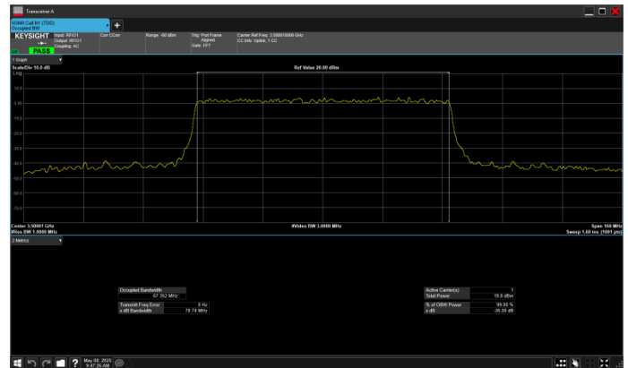
n78_1_80MHz_30kHz_3500MHz_DFT-s-OFDM \pi/2 BPSK_RB216@0
