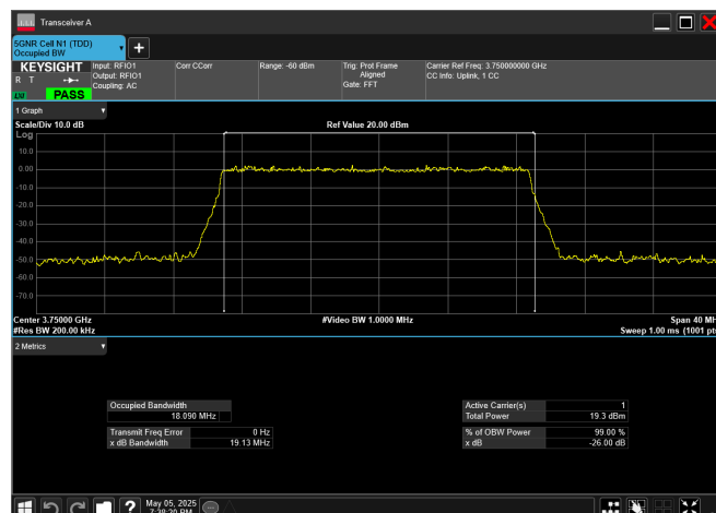
n78_3_20MHz_30kHz_3750MHz_DFT-s-OFDM 64 QAM_RB50@0
