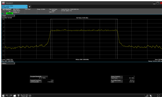
n78_1_70MHz_30kHz_3500MHz_CP-OFDM 256 QAM_RB189@0
