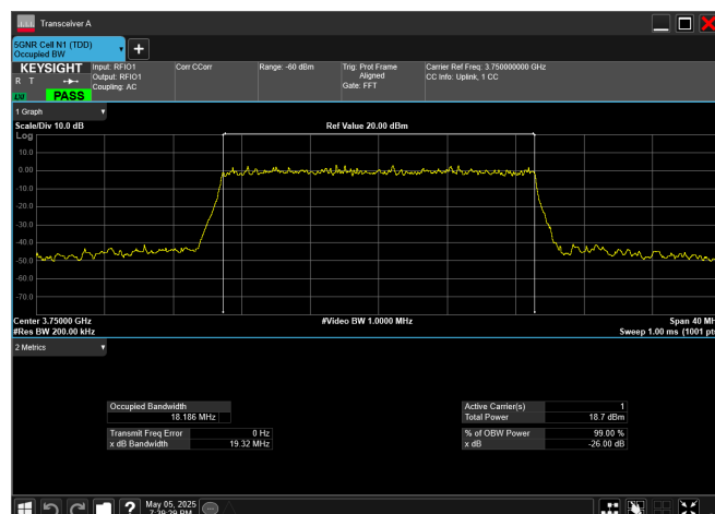
n78_3_20MHz_30kHz_3750MHz_CP-OFDM QPSK_RB51@0
