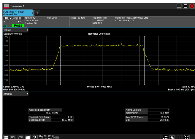
n78_3_20MHz_30kHz_3750MHz_DFT-s-OFDM 256 QAM_RB50@0
