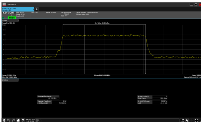
n78_1_80MHz_30kHz_3500MHz_DFT-s-OFDM QPSK_RB216@0
