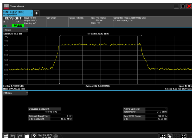
n78_3_20MHz_30kHz_3750MHz_DFT-s-OFDM 16 QAM_RB50@0
