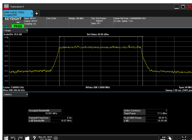
n77_3_20MHz_30kHz_3840MHz_DFT-s-OFDM 256 QAM_RB50@0
