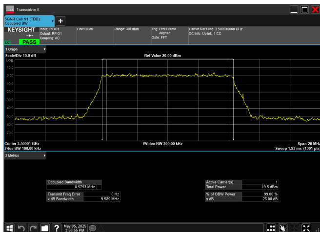
n78_1_10MHz_30kHz_3500MHz_CP-OFDM QPSK_RB24@0
