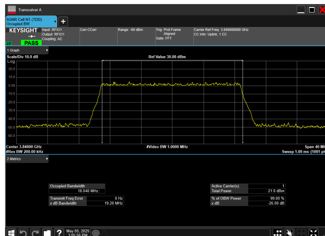
n77_3_20MHz_30kHz_3840MHz_DFT-s-OFDM 64 QAM_RB50@0
