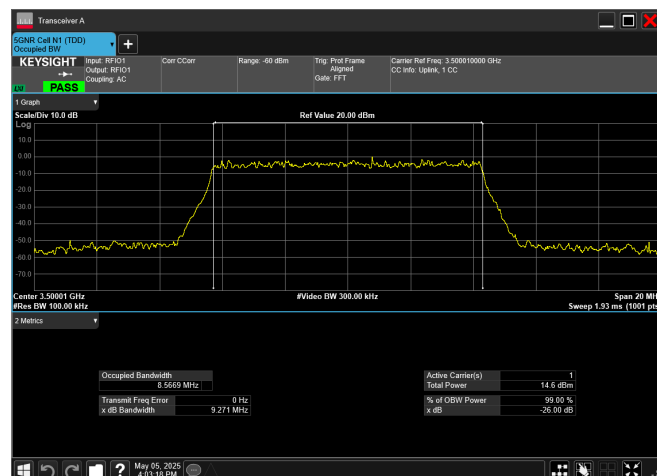
n78_1_10MHz_30kHz_3500MHz_CP-OFDM 256 QAM_RB24@0
