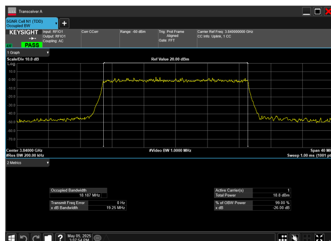
n77_3_20MHz_30kHz_3840MHz_CP-OFDM QPSK_RB51@0
