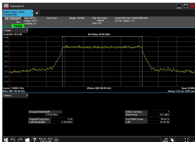
n78_1_10MHz_30kHz_3500MHz_CP-OFDM 64 QAM_RB24@0
