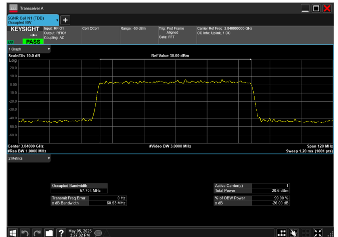
n77_3_60MHz_30kHz_3840MHz_CP-OFDM QPSK_RB162@0
