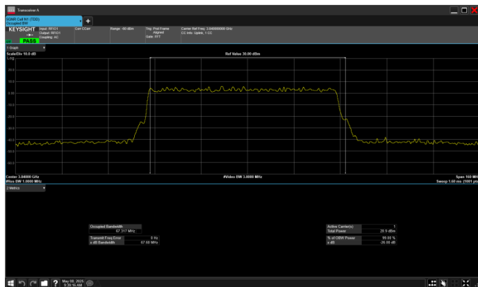
n77_3_70MHz_30kHz_3840MHz_CP-OFDM QPSK_RB189@0
