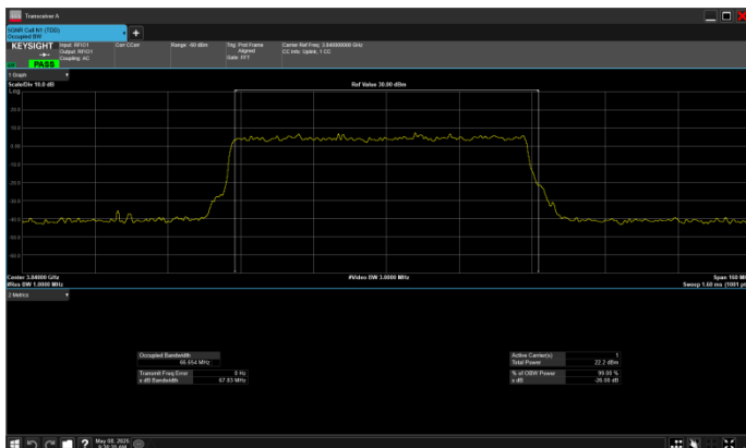
n77_3_70MHz_30kHz_3840MHz_DFT-s-OFDM QPSK_RB180@0
