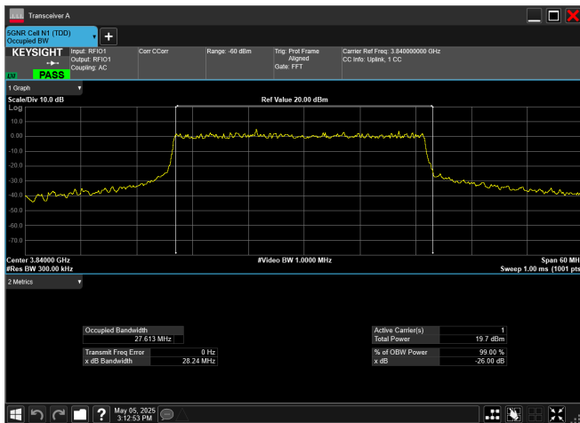
n77_3_30MHz_30kHz_3840MHz_CP-OFDM QPSK_RB78@0
