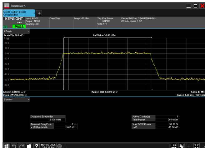
n77_3_20MHz_30kHz_3840MHz_DFT-s-OFDM 256 QAM_RB50@0
