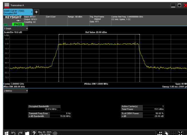
n77_3_20MHz_30kHz_3840MHz_CP-OFDM QPSK_RB51@0
