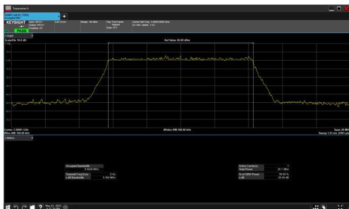
n77_1_10MHz_30kHz_3500MHz_CP-OFDM QPSK_RB24@0
