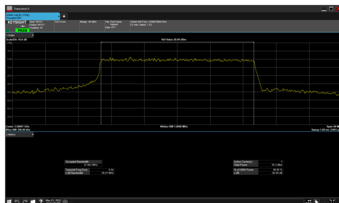
n77_1_30MHz_30kHz_3500MHz_CP-OFDM QPSK_RB78@0
