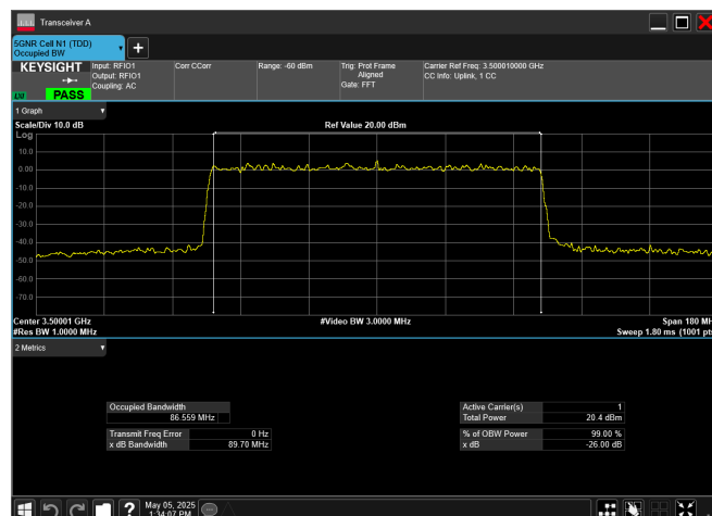
n77_1_90MHz_30kHz_3500MHz_CP-OFDM QPSK_RB245@0
