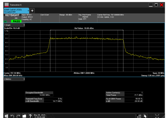
n12_15MHz_15kHz_707.5MHz_CP-OFDM QPSK_RB79@0
