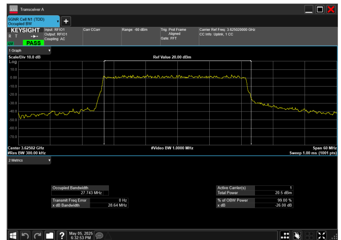
n78_2_30MHz_30kHz_3625MHz_DFT-s-OFDM 64 QAM_RB75@0
