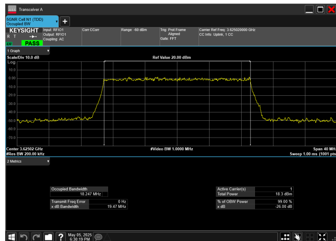
n78_2_20MHz_30kHz_3625MHz_CP-OFDM 256 QAM_RB51@0
