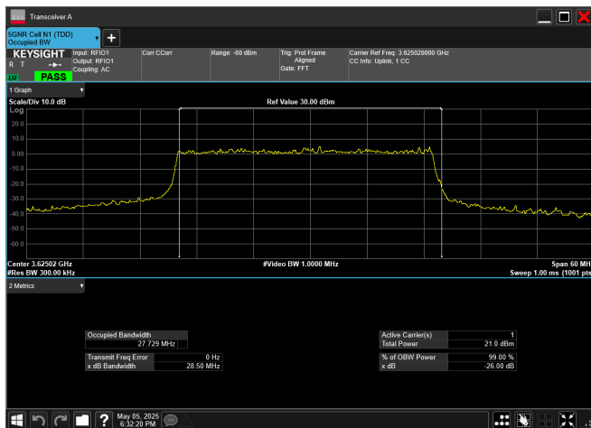
n78_2_30MHz_30kHz_3625MHz_DFT-s-OFDM 16 QAM_RB75@0
