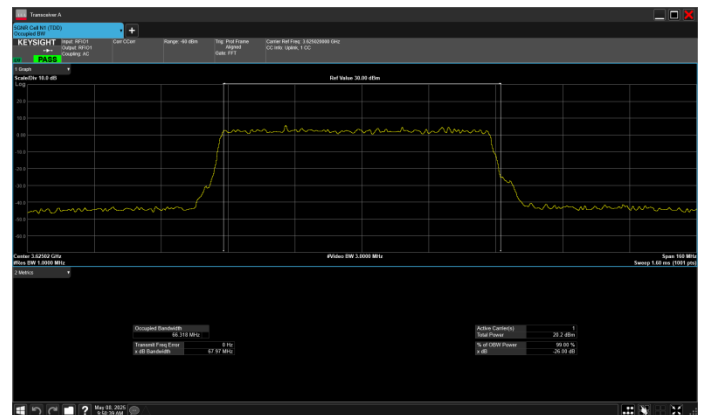
n78_2_70MHz_30kHz_3625MHz_CP-OFDM QPSK_RB189@0
