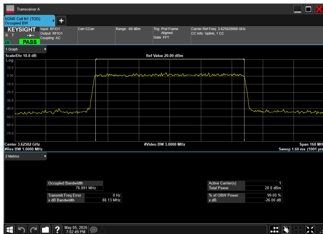
n78_2_80MHz_30kHz_3625MHz_CP-OFDM QPSK_RB217@0
