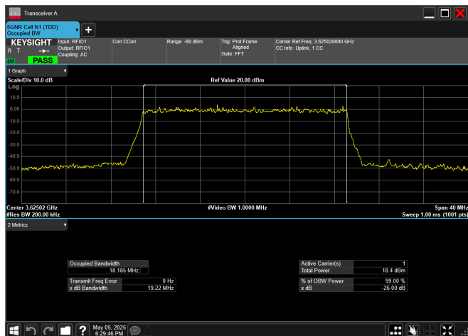
n78_2_20MHz_30kHz_3625MHz_CP-OFDM 64 QAM_RB51@0
