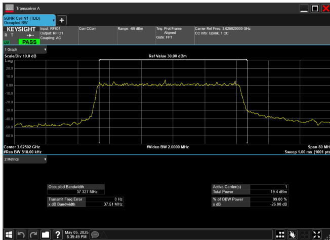
n78_2_40MHz_30kHz_3625MHz_CP-OFDM QPSK_RB106@0
