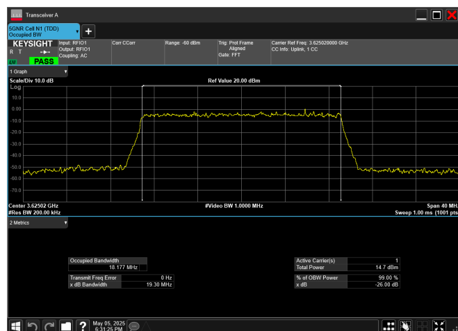
n78_2_20MHz_30kHz_3625MHz_CP-OFDM 256 QAM_RB51@0
