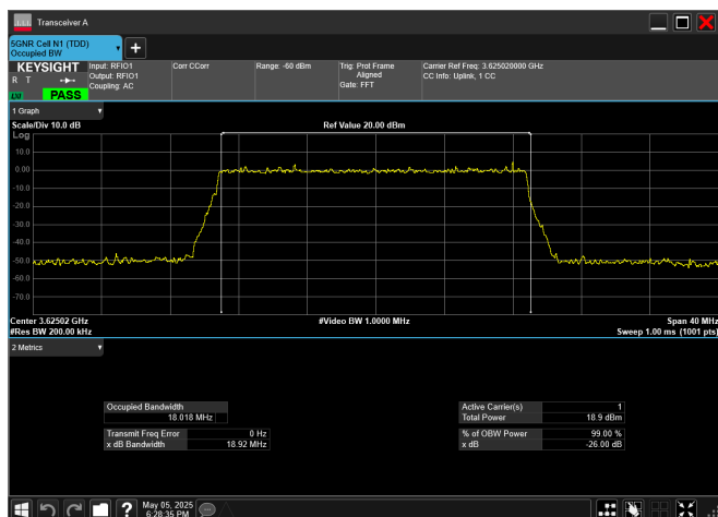
n78_2_20MHz_30kHz_3625MHz_CP-OFDM QPSK_RB51@0
