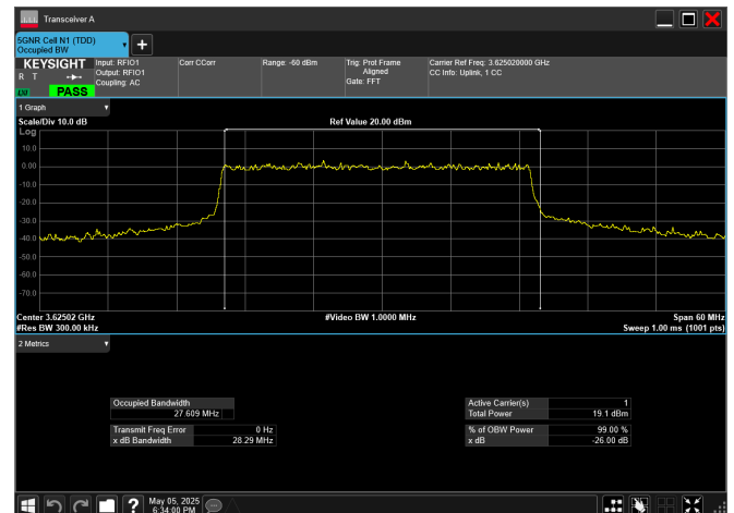
n78_2_30MHz_30kHz_3625MHz_CP-OFDM QPSK_RB78@0
