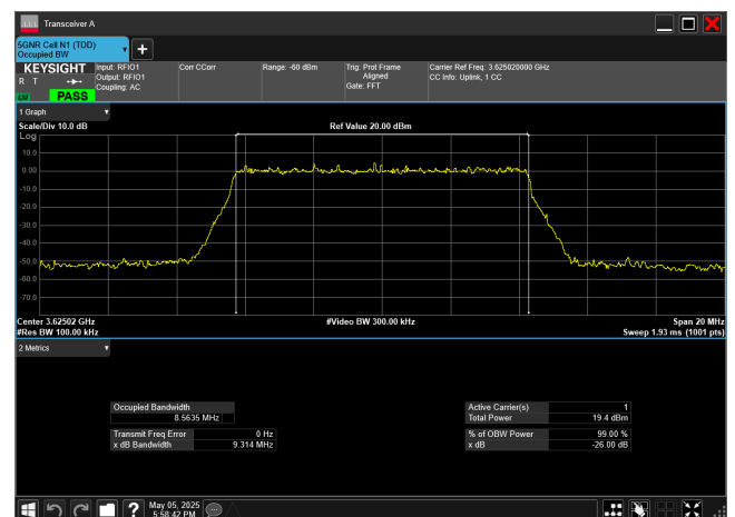
n78_2_10MHz_30kHz_3625MHz_DFT-s-OFDM 16 QAM_RB24@0
