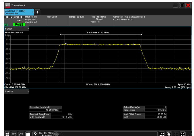
n77_2_20MHz_30kHz_3625MHz_CP-OFDM QPSK_RB51@0
