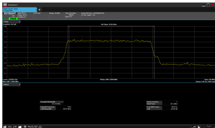
n77_2_70MHz_30kHz_3625MHz_CP-OFDM QPSK_RB189@0
