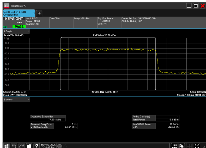
n77_2_90MHz_30kHz_3625MHz_DFT-s-OFDM QPSK_RB243@0
