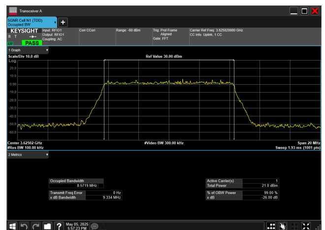
n78_2_10MHz_30kHz_3625MHz_DFT-s-OFDM 16 QAM_RB24@0
