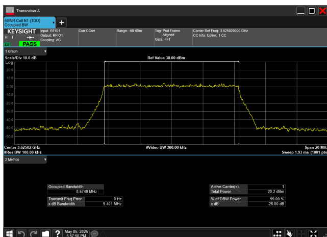
n78_2_10MHz_30kHz_3625MHz_DFT-s-OFDM QPSK_RB24@0
