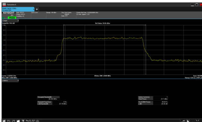
n77_2_70MHz_30kHz_3625MHz_DFT-s-OFDM QPSK_RB180@0
