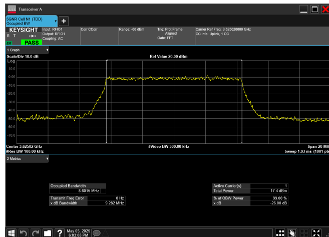
n78_2_10MHz_30kHz_3625MHz_CP-OFDM 256 QAM_RB24@0
