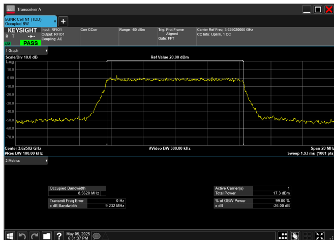
n78_2_10MHz_30kHz_3625MHz_CP-OFDM 64 QAM_RB24@0
