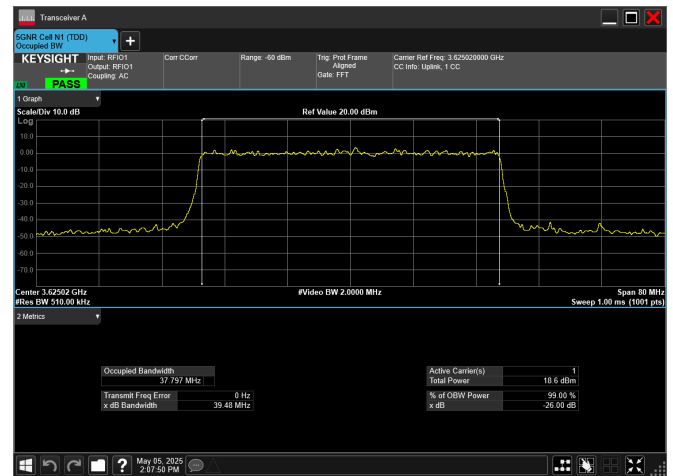
n77_2_50MHz_30kHz_3625MHz_DFT-s-OFDM \pi/2 BPSK_RB128@0
