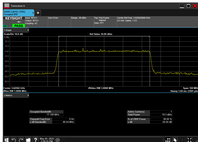
n77_2_90MHz_30kHz_3625MHz_DFT-s-OFDM \pi/2 BPSK_RB243@0
