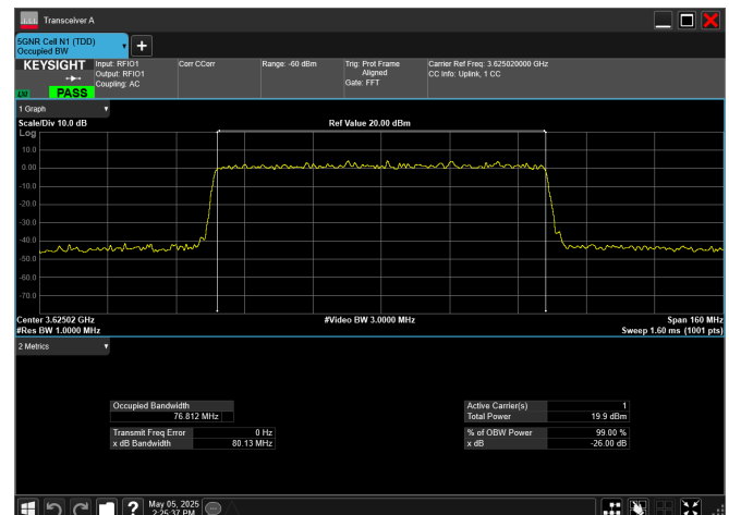
n77_2_80MHz_30kHz_3625MHz_CP-OFDM QPSK_RB217@0
