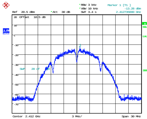
802.11b_2412MHz_Chain 0
