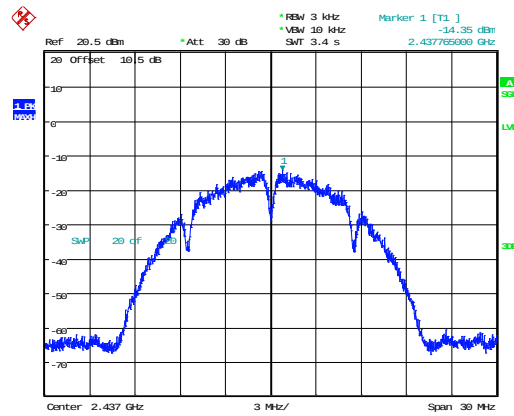
802.11b_2437MHz_Chain 0
