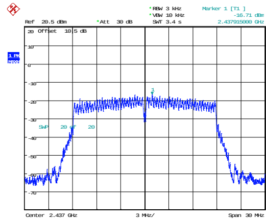
802.11n20_2437MHz_Chain 0
