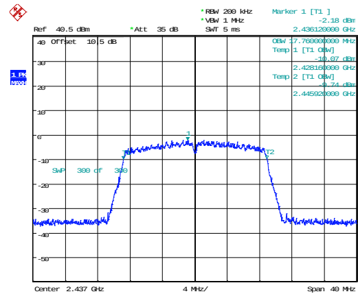
802.11n20_2437MHz_Chain 0
