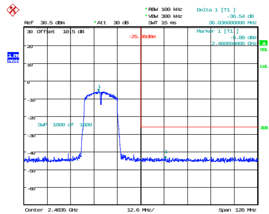
802.11n20_2462MHz_Chain 0
