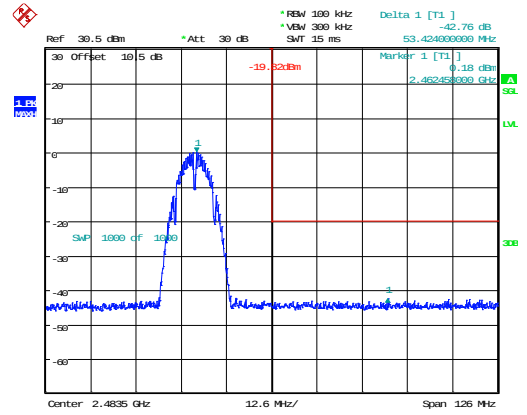
802.11b_2462MHz_Chain 0
