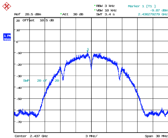
802.11b_2437MHz_Chain 1
