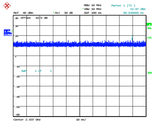
802.11n20_2437MHz_Chain 0
