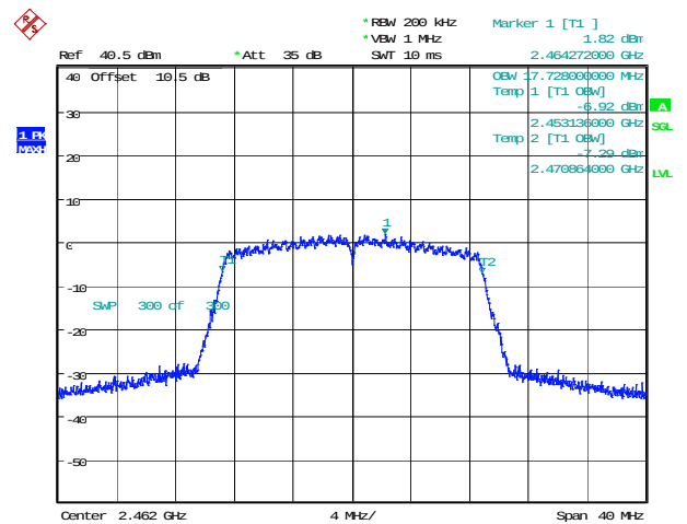
802.11n20_2462MHz_Chain 1
