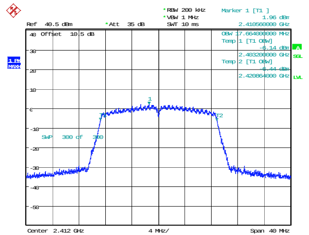
802.11n20_2412MHz_Chain 1
