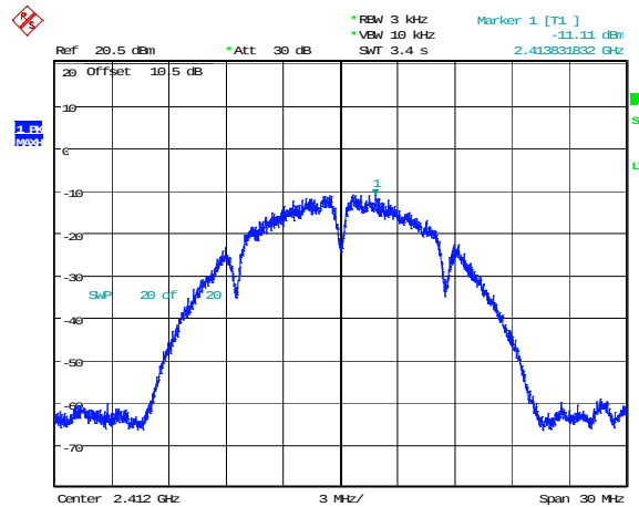
802.11b_2412MHz_Chain 1
