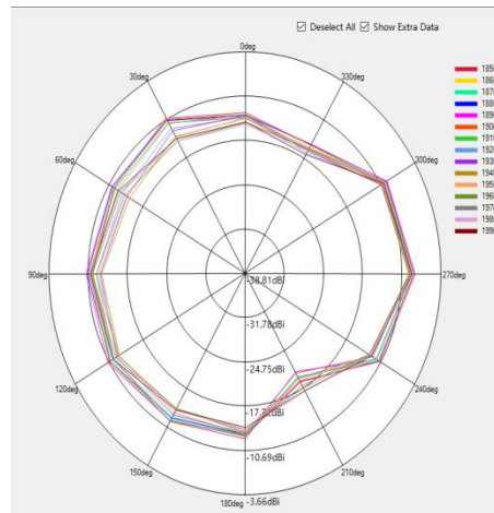
LTEB2 Theta=90deg
