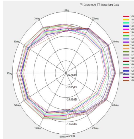
GPS Theta=90deg
