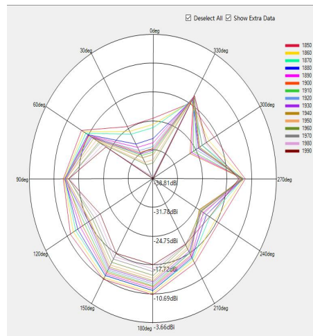
LTEB2 Phi=0deg
