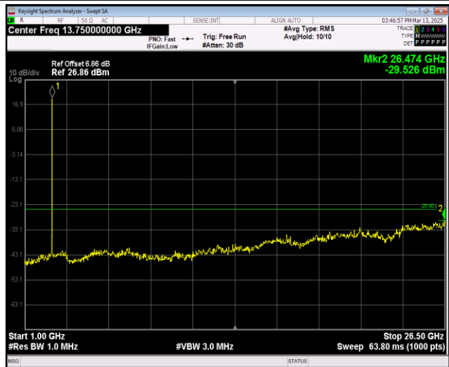
Band41-5MHz-64QAM-40065-1RB#0-Range2:1000~26500MHz
