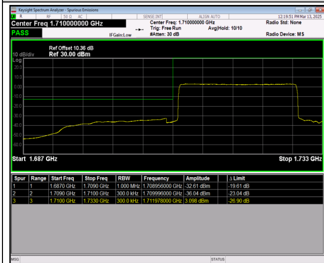
Band4-20MHz-QPSK-20300-1RB#99
