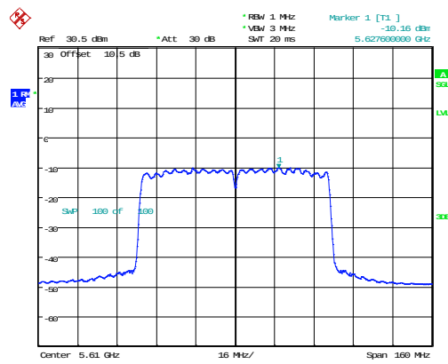
802.11ac80_5610MHz
