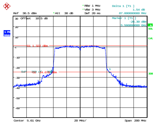
802.11ac80_5610MHz
