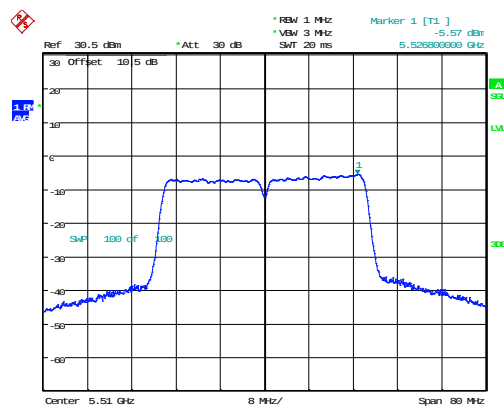
802.11n40_5510MHz
