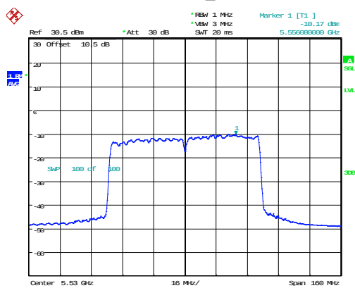
802.11ac80_5530MHz
