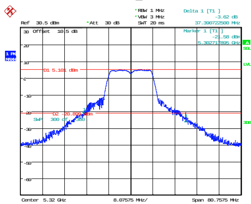
802.11a_5320MHz
