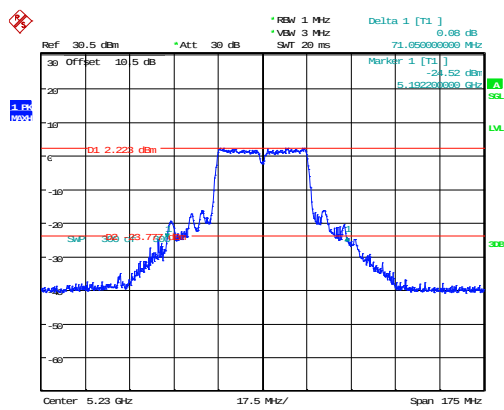
802.11n40_5230MHz
