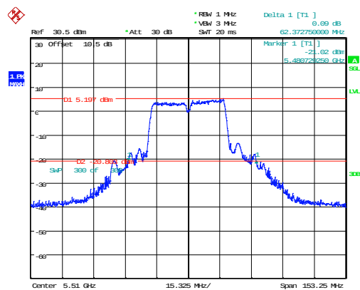
802.11n40_5510MHz
