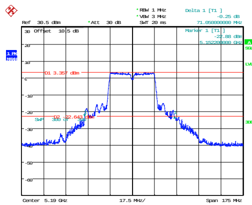
802.11n40_5190MHz
