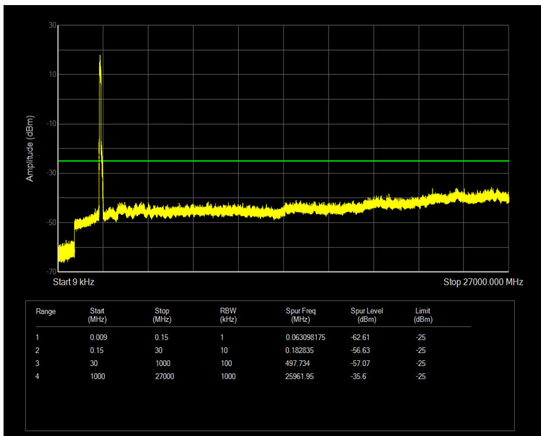
n41 SCS=30kHz DFT_QPSK BW=100MHz Channel=509202 RB=1@0
