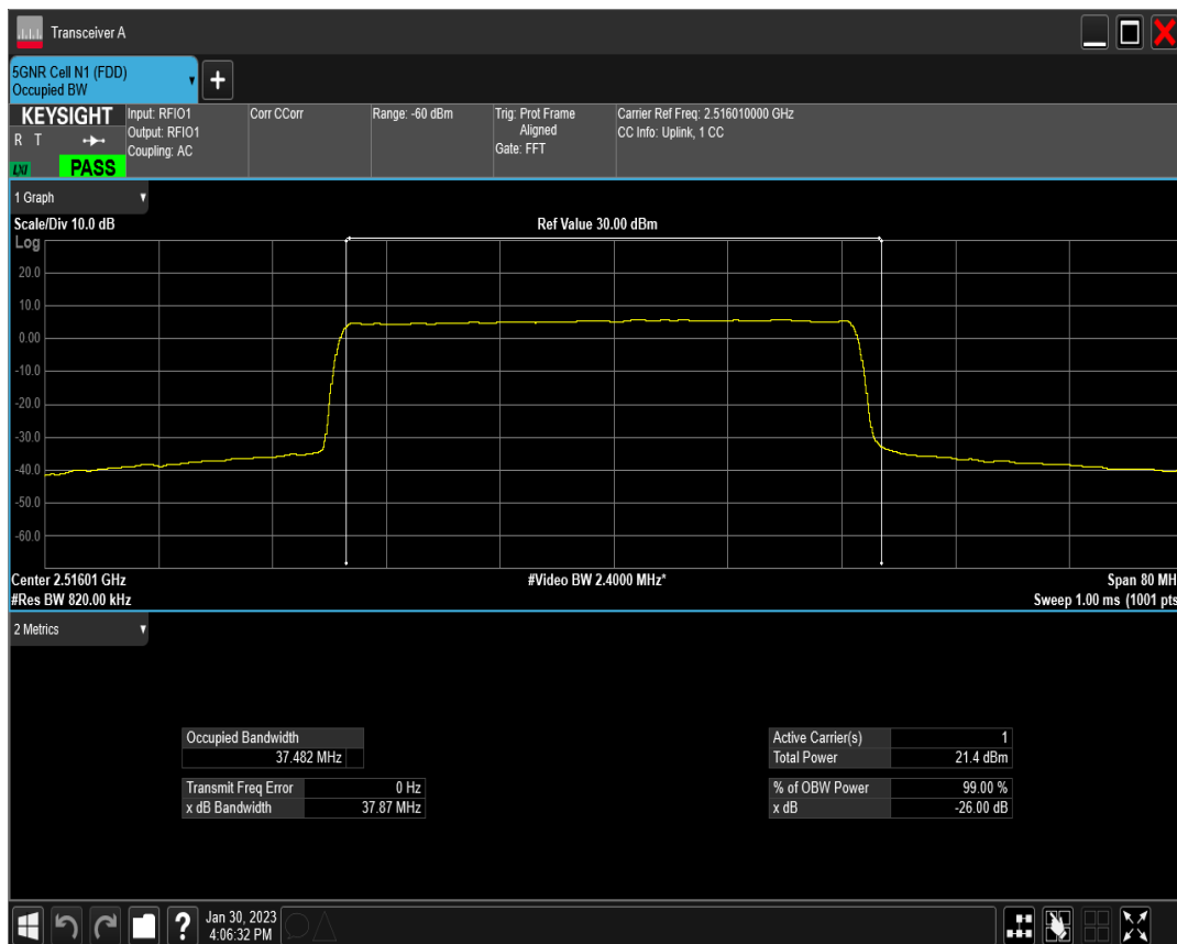
n41 SCS=30kHz CP_QPSK BW=40MHz Channel=503202 RB=106@0
