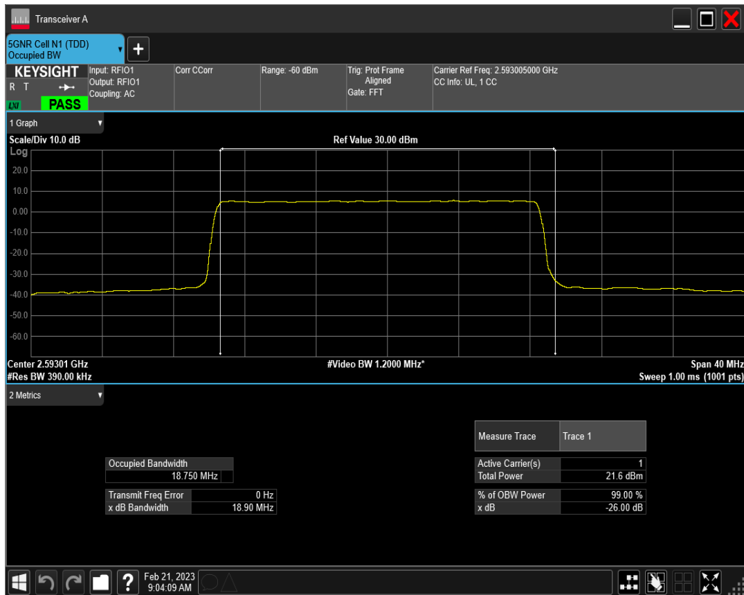
n41 SCS=15kHz CP_QPSK BW=20MHz Channel=518601 RB=106@0
