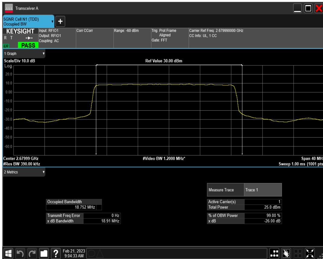
n41 SCS=15kHz DFT_QPSK BW=20MHz Channel=535998 RB=100@0
