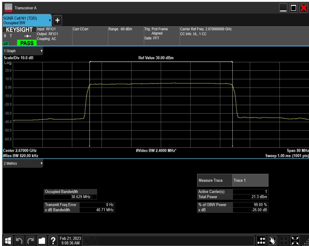
n41 SCS=15kHz CP_QPSK BW=40MHz Channel=534000 RB=216@0
