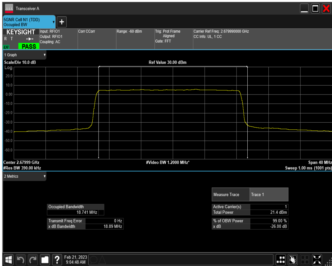
n41 SCS=15kHz CP_QPSK BW=20MHz Channel=535998 RB=106@0
