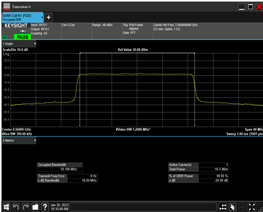
n7 SCS=30kHz CP_QPSK BW=20MHz Channel=512000 RB=51@0
