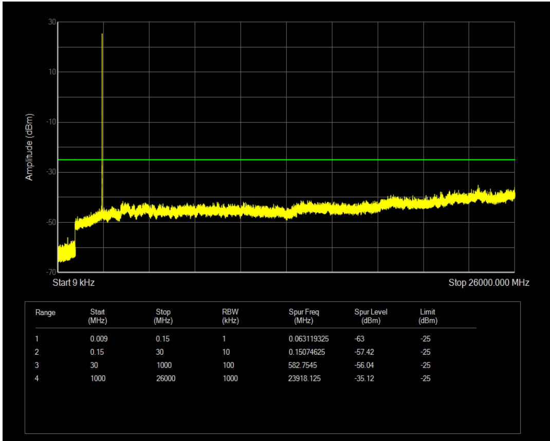
n7 SCS=30kHz DFT_QPSK BW=10MHz Channel=513000 RB=1@0
