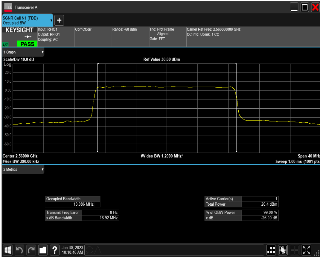
n7 SCS=30kHz DFT_QAM256 BW=20MHz Channel=512000 RB=50@0
