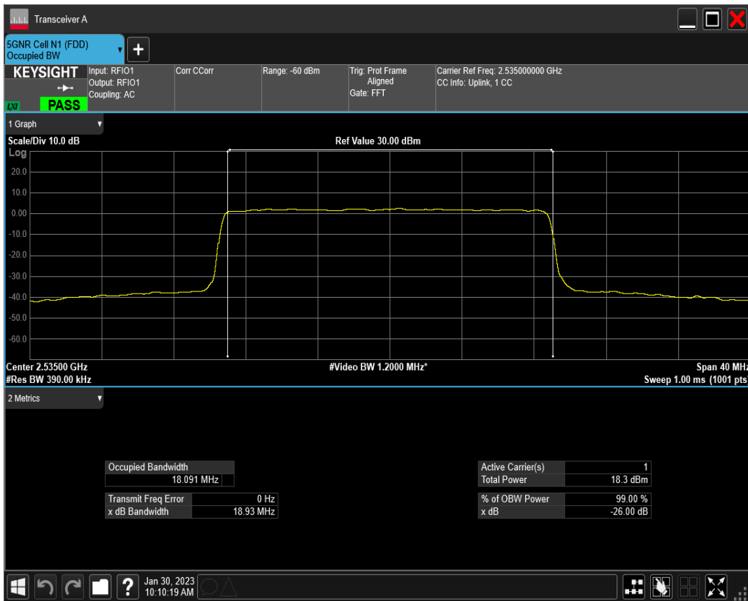
n7 SCS=30kHz CP_QPSK BW=20MHz Channel=507000 RB=51@0
