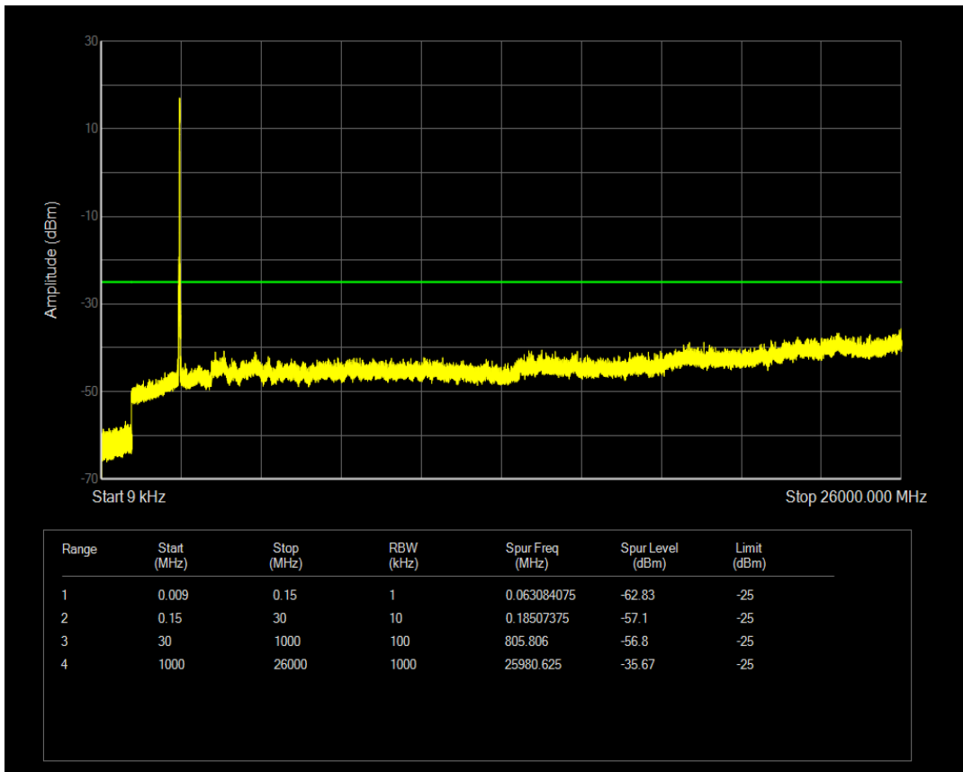
n7 SCS=30kHz DFT_QPSK BW=20MHz Channel=512000 RB=1@0
