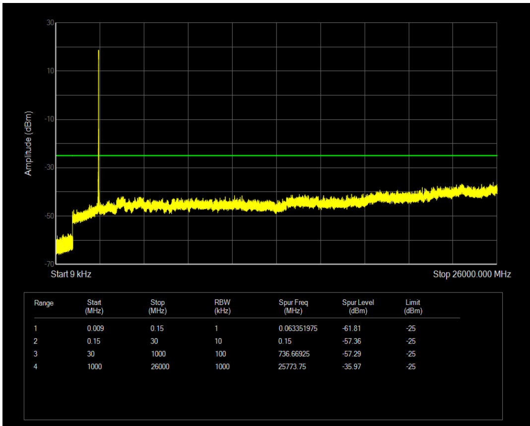
n7 SCS=30kHz DFT_QPSK BW=10MHz Channel=507000 RB=1@0
