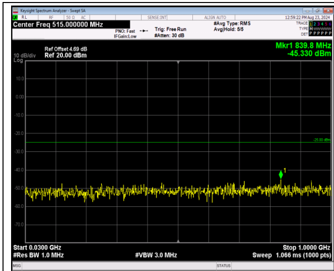
Band41-20MHz-QPSK-41140-1RB#0-Range1:30~100 0MHz
