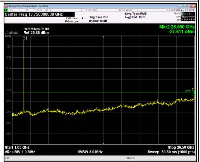
Band41-5MHz-QPSK-41215-1RB#0-Range2:1000~2 6500MHz
