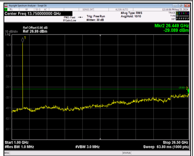
Band41-5MHz-QPSK-41215-1RB#0-Range2:1000~2 6500MHz
