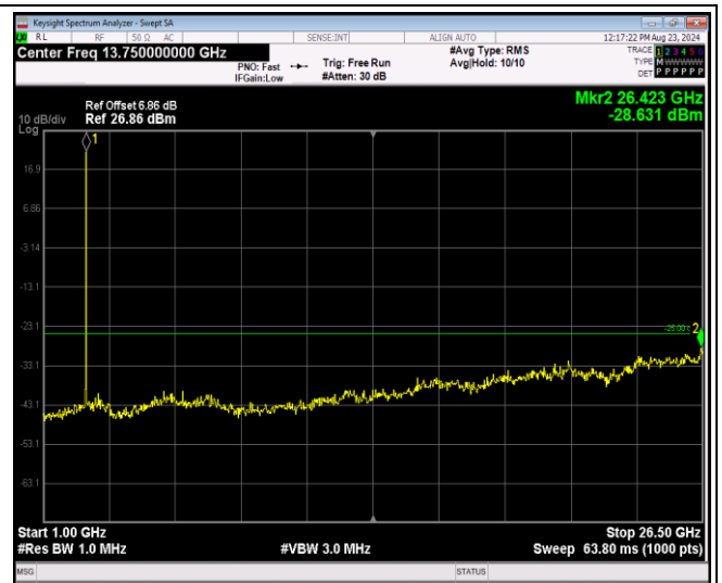
Band41-5MHz-64QAM-40065-1RB#0-Range2:1000~ 26500MHz
