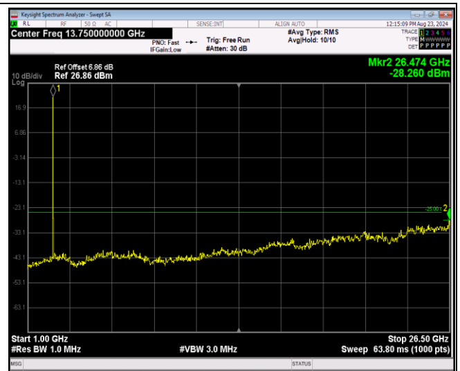
Band41-5MHz-QPSK-40640-1RB#0-Range2:1000~2 6500MHz
