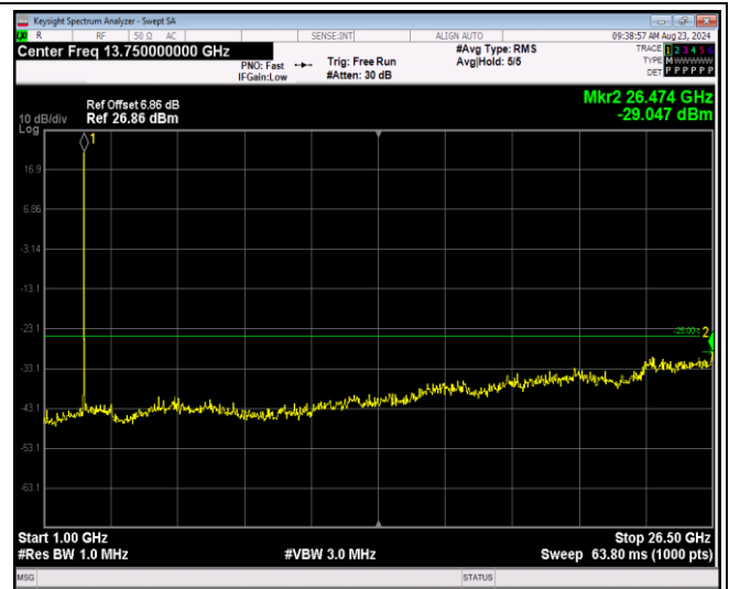
Band7-20MHz-16QAM-21350-1RB#0-Range2:1000~ 26500MHz
