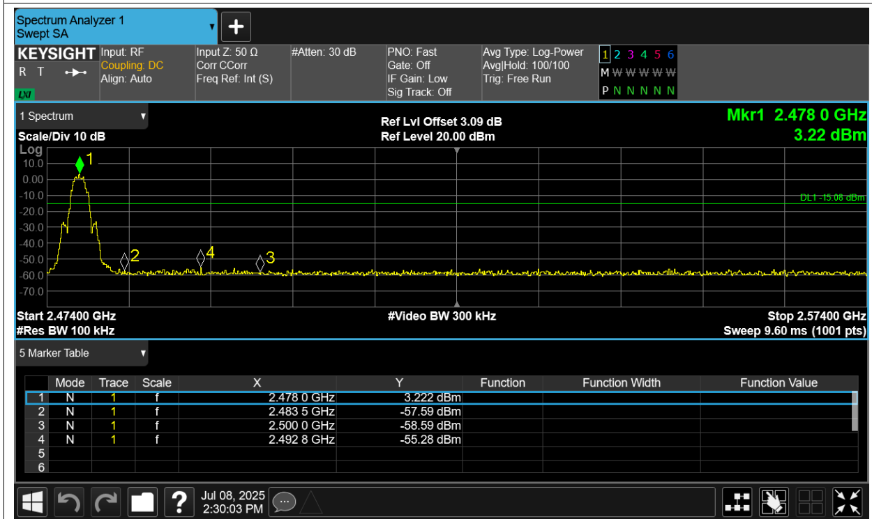
Band Edge NVNT BLE 2478MHz Ant3 Emission
