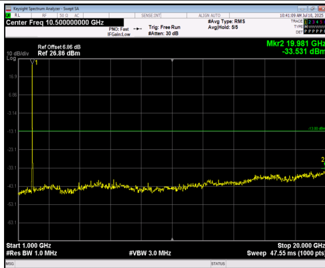
Band25-20MHz-QPSK-26590-1RB#0-Range2:1000~20000MHz
