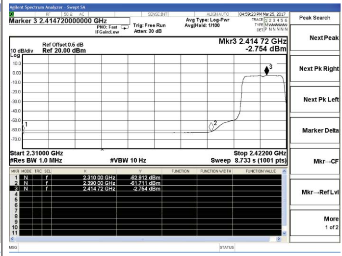
802.11g-Low channel(Average)
