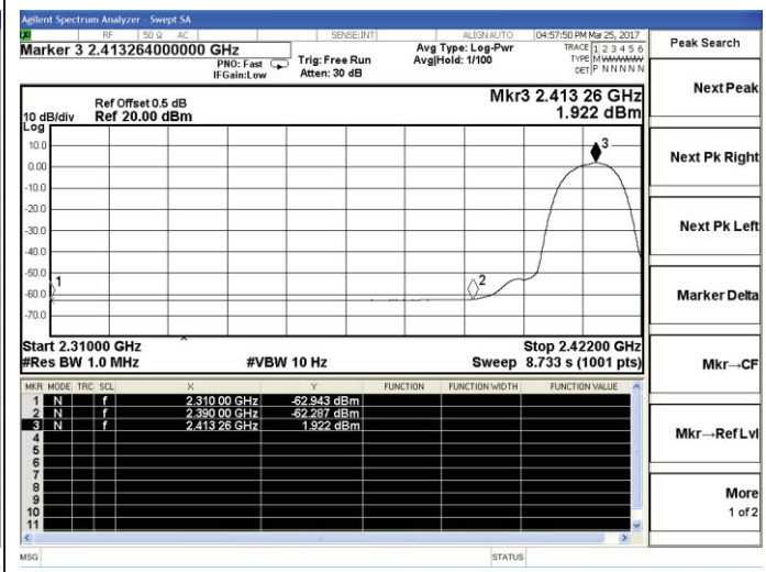
802.11b-Low channel(Average)
