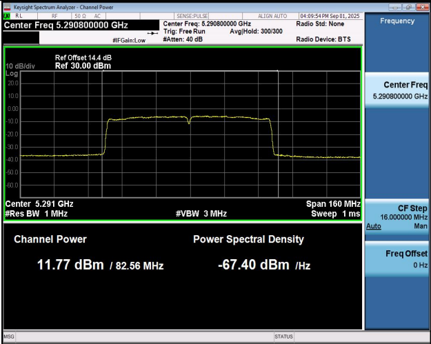
11AC80SISO-Ant1-5290-PASS
