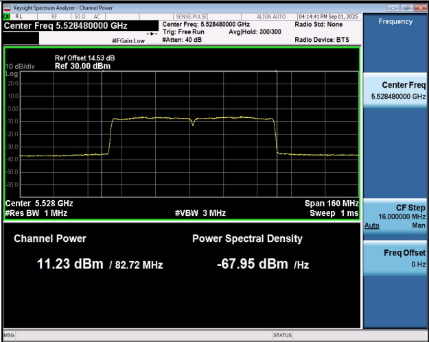
11AC80SISO-Ant1-5530-PASS
