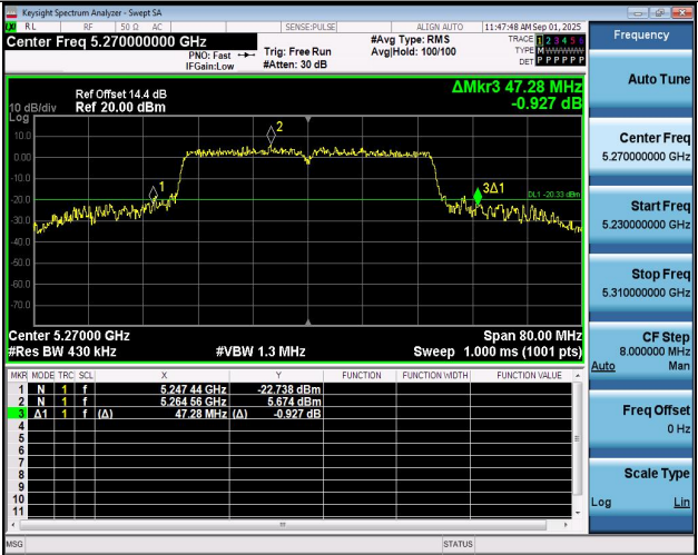
11N40SISO-Ant1-5270
