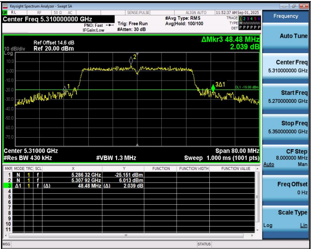
11N40SISO-Ant1-5310
