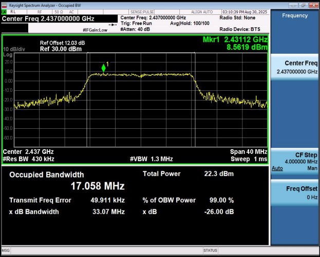
11G-Ant1-2437
