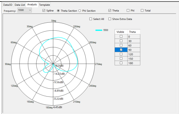
G/W/B: 5500Mhz
