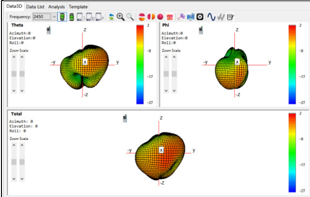
G/W/B: 2450Mhz
