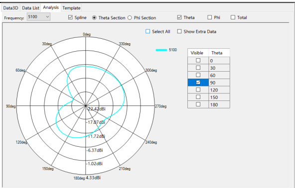
G/W/B:5100Mhz
