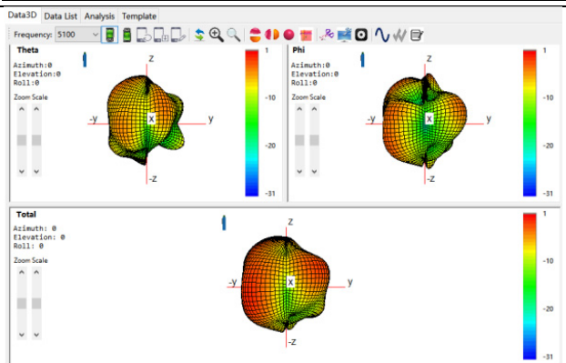
G/W/B: 5100Mhz
