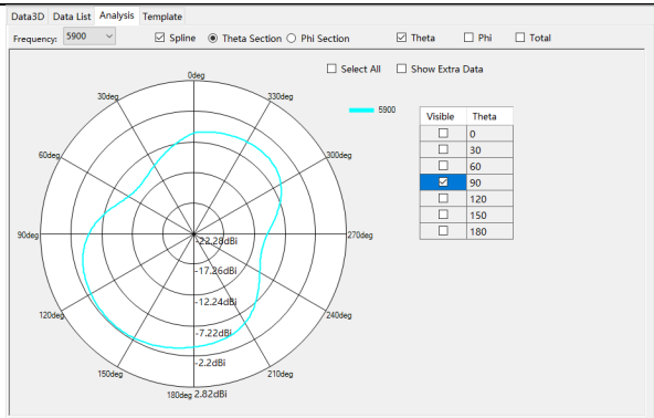
G/W/B:5900Mhz
