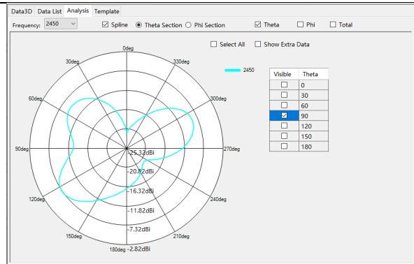
G/W/B: 2450Mhz
