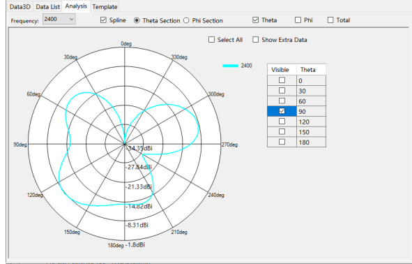
G/W/B: 2400Mhz
