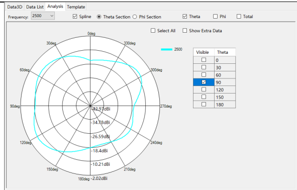
G/W/B: 2500Mhz
