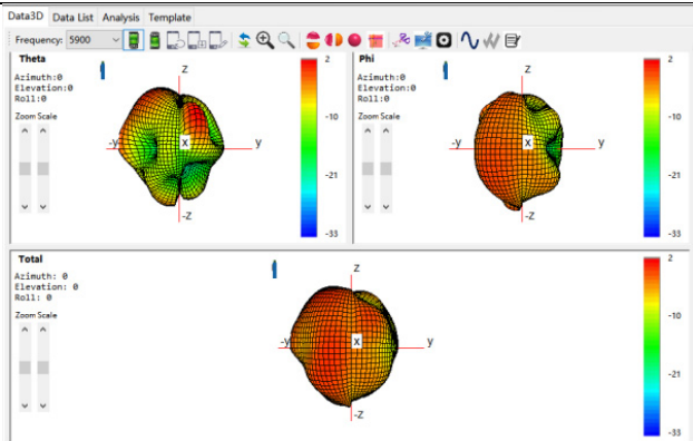
G/W/B: 5900Mhz
