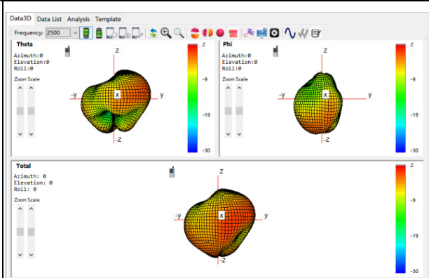
G/W/B: 2500Mhz
