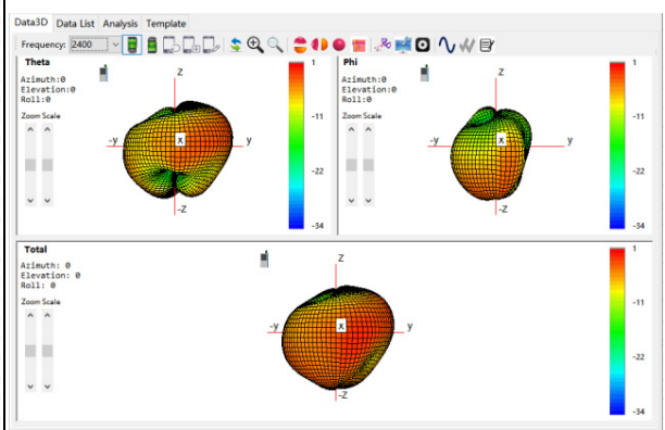
G/W/B: 2400Mhz
