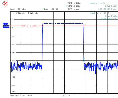
DH1_Hopping 0.385ms
