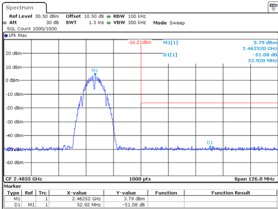
802.11b_2462MHz
