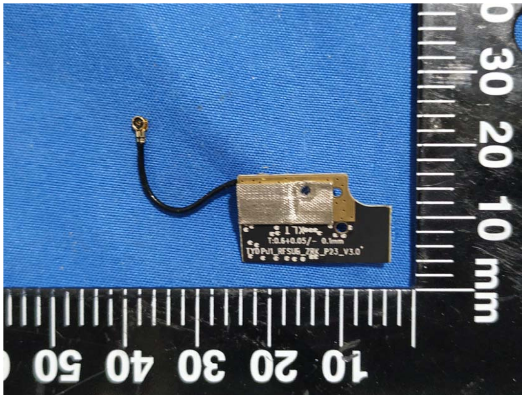
GPS ANT
