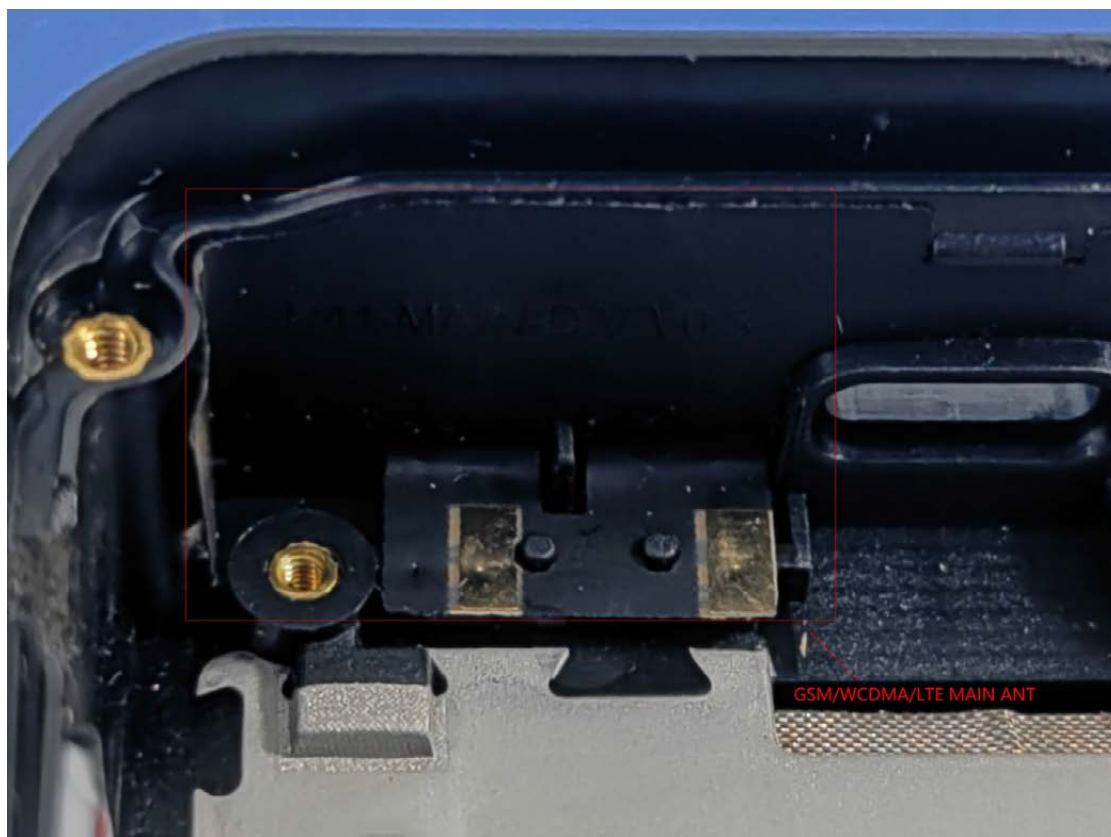
GSM/WCDMA/LTE MIAN ANT
