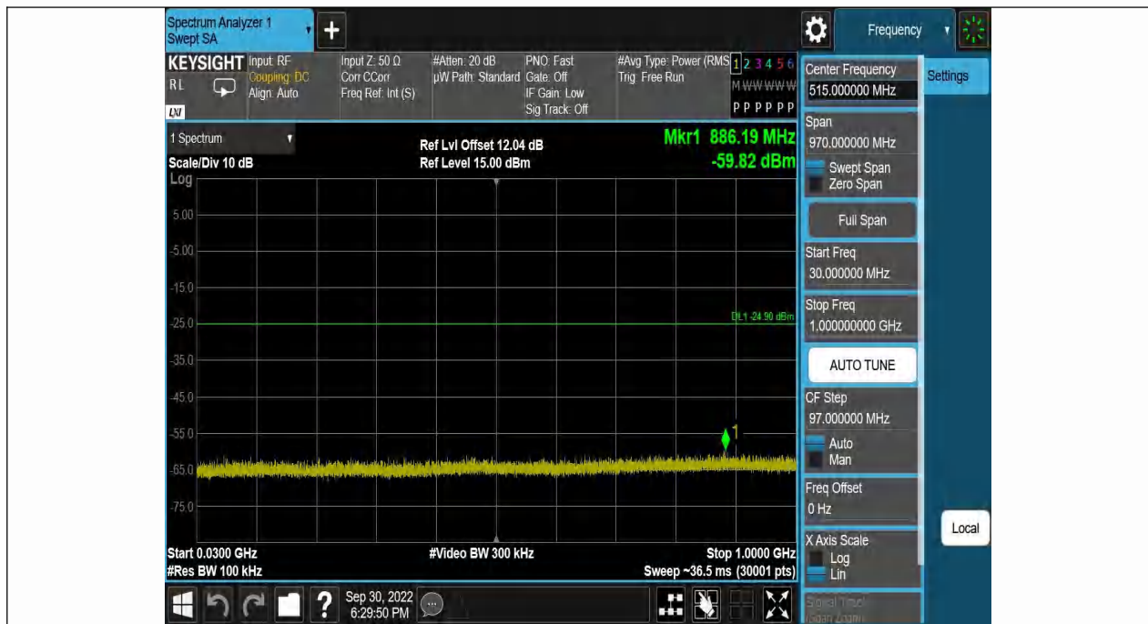
BLE 2M-Ant1-2480-30~1000--4.90
