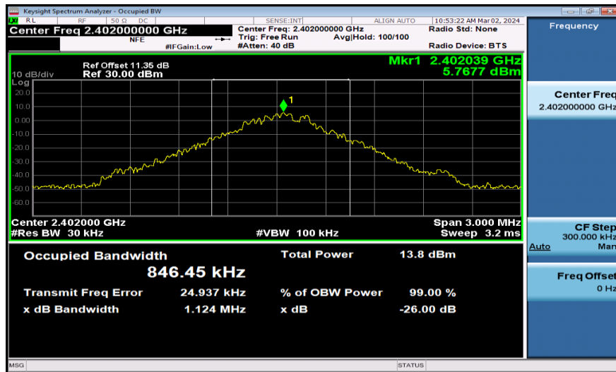
DH5-Ant1-2402
