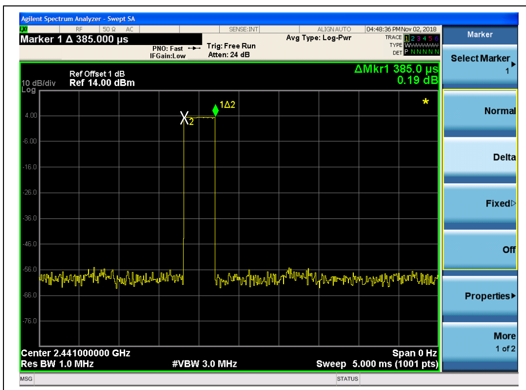
(DH1, GFSK)
