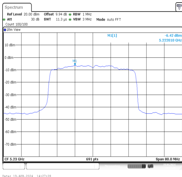
11AX40MIMO-Ant1-5230-PASS
