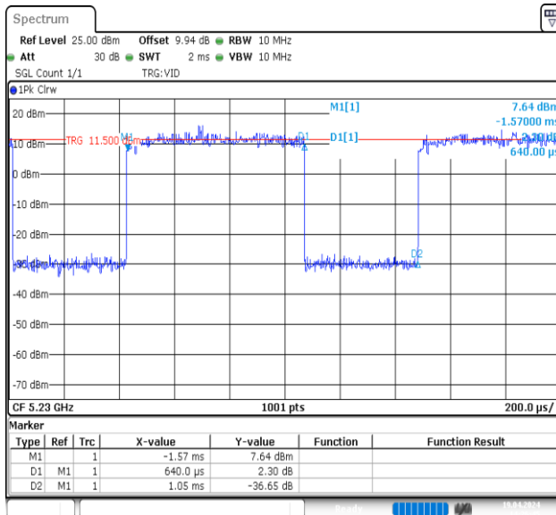
NTVN-11AX40MIMO-Ant1-5230
