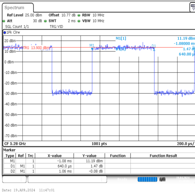
NTVN-11AX20MIMO-Ant1-5280
