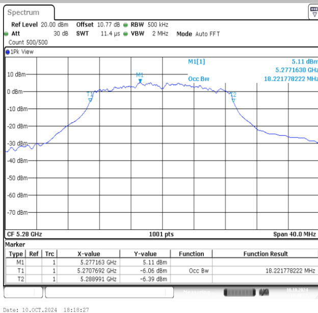
11AC20MIMO-Ant1-5280
