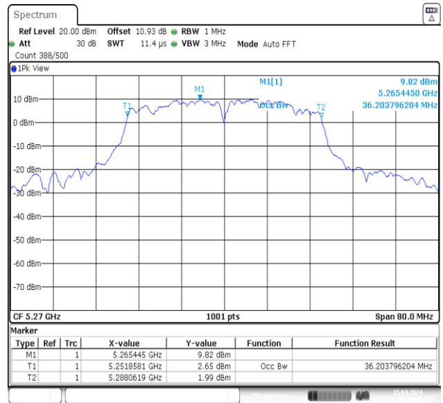
11N40MIMO-Ant2-5270
