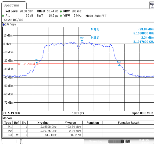
11N40MIMO-Ant1-5190
