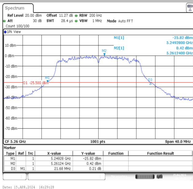
11N20MIMO-Ant1-5260
