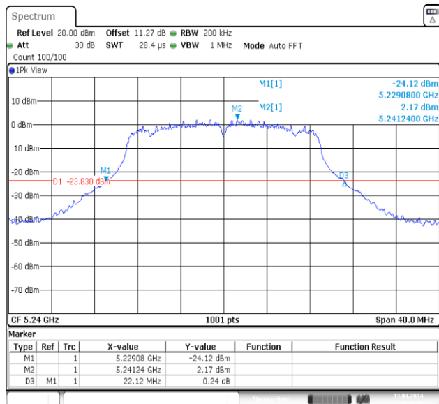
11N20MIMO-Ant1-5240
