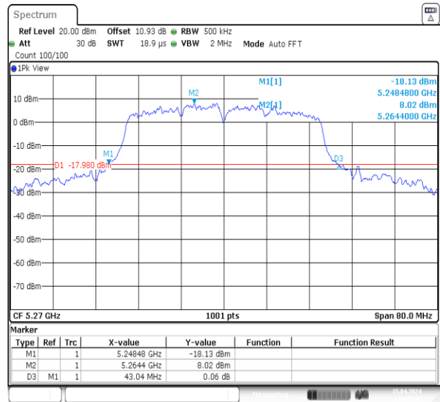
11N40MIMO-Ant2-5270
