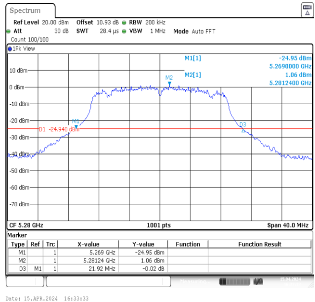
11N20MIMO-Ant2-5280
