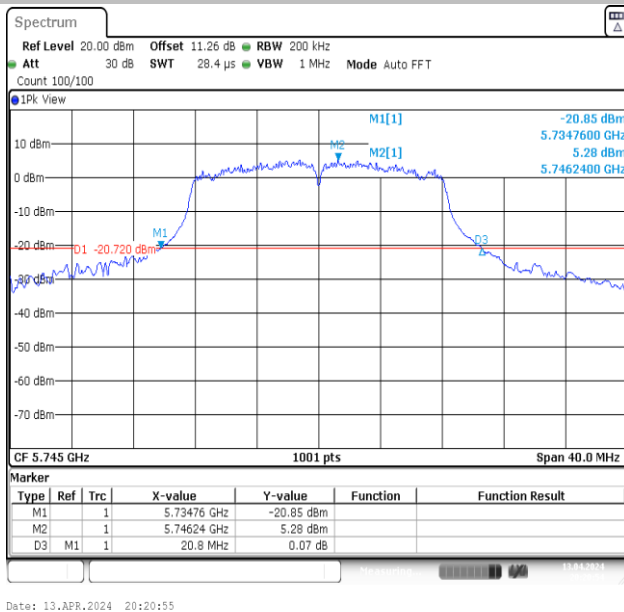
11A-Ant1-5745
