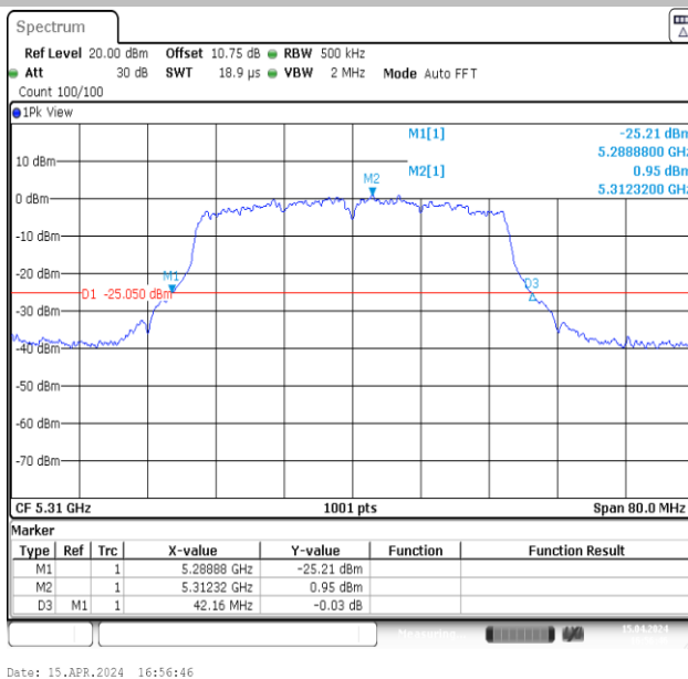
11N40MIMO-Ant1-5310
