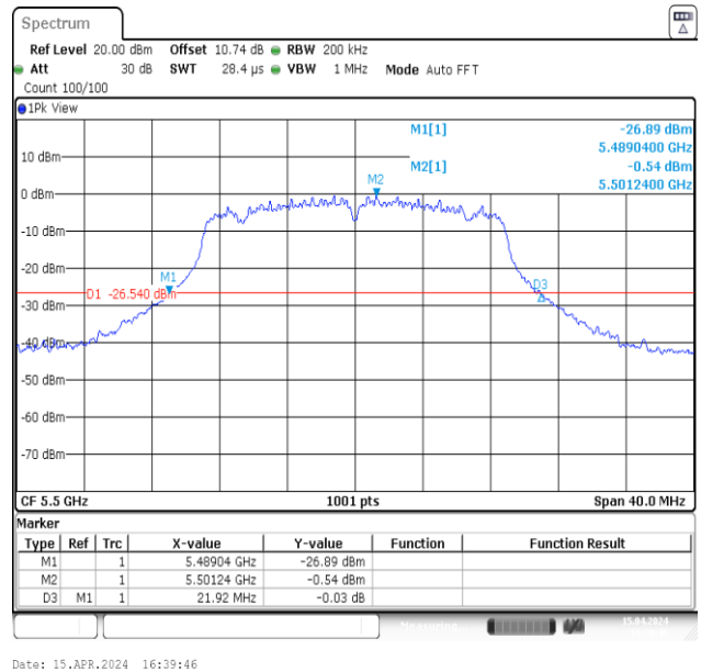
11N20MIMO-Ant2-5500
