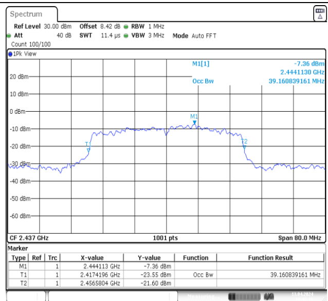
11AX40MIMO-Ant2-2437
