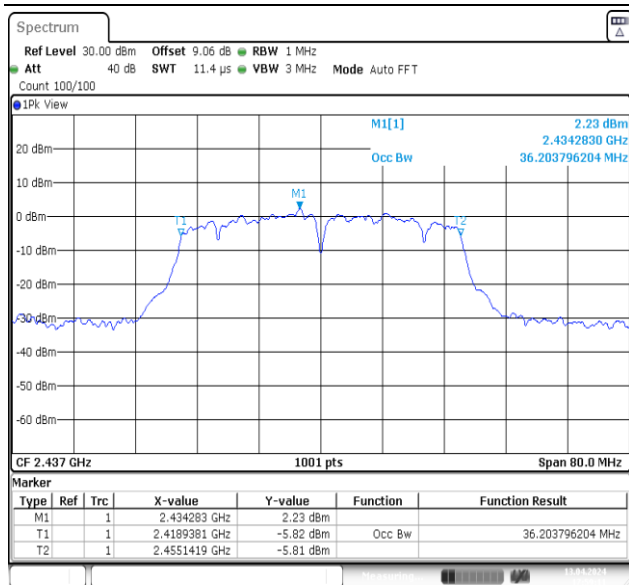
11N40MIMO-Ant1-2437
