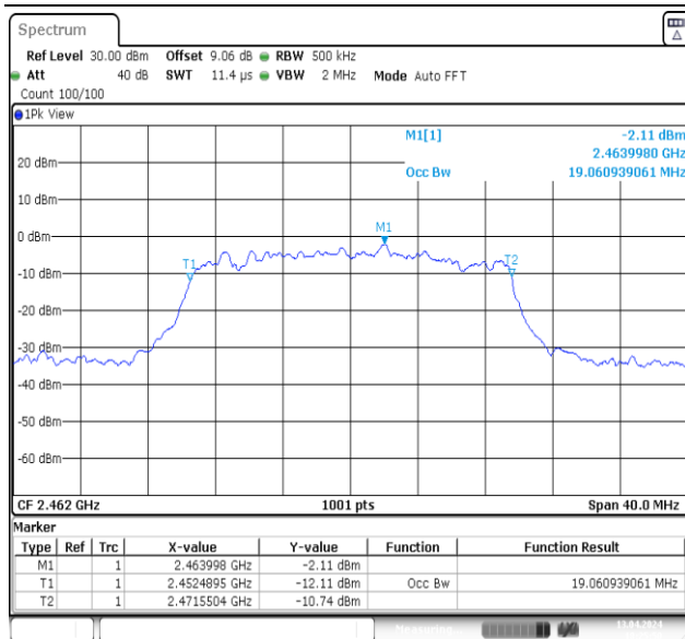
11AX20MIMO-Ant1-2462
