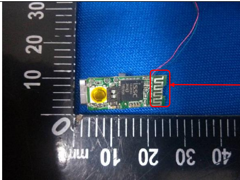
Antenna
