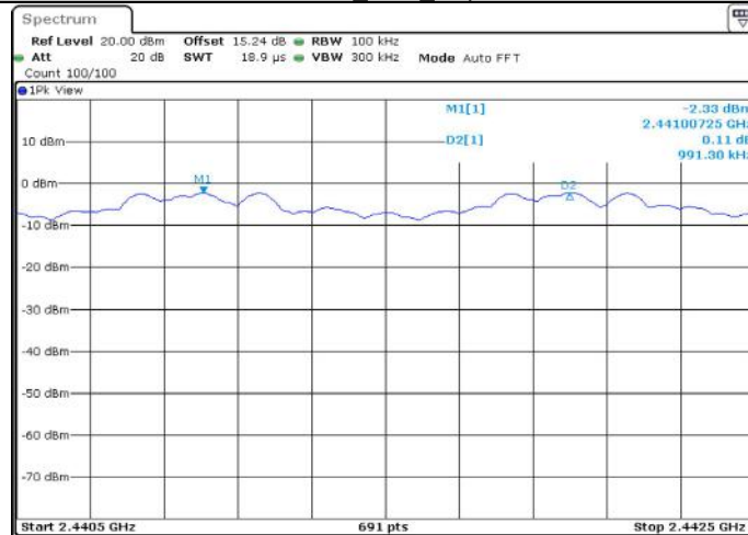
2DH1_Ant1_Hop
