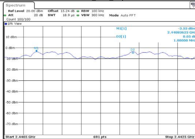
3DH1_Ant1_Hop
