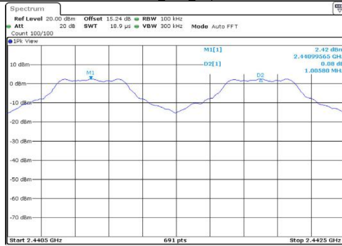
DH1_Ant1_Hop
