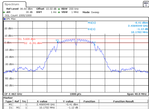
802.11b_2462MHz_Chain 1
