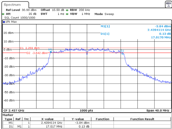
802.11n20_2437MHz_Chain 1
