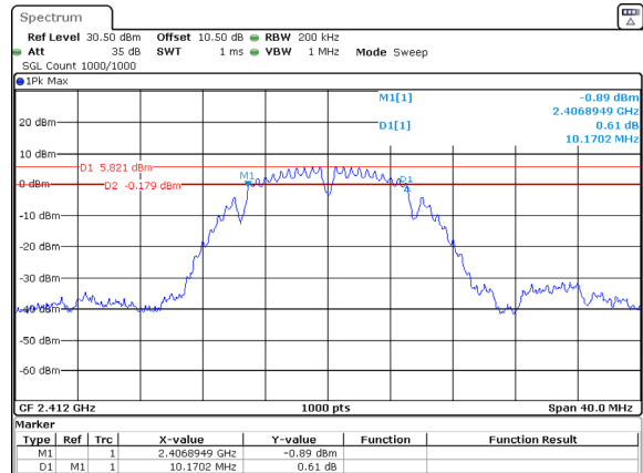
802.11b_2412MHz_Chain 1
