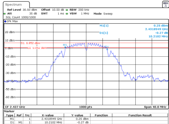
802.11b_2437MHz_Chain 0
