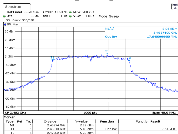
802.11n20_2462MHz_Chain 1
