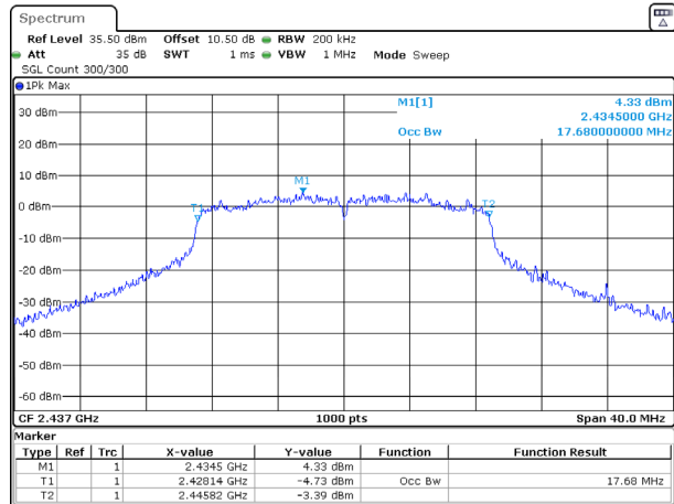
802.11n20_2437MHz_Chain 0
