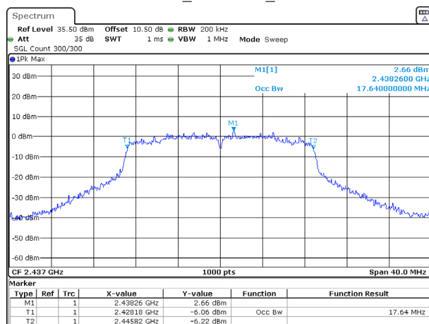
802.11n20_2437MHz_Chain 1
