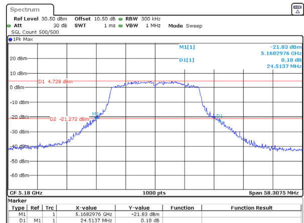
802.11ac20_5180MHz_Chain 1
