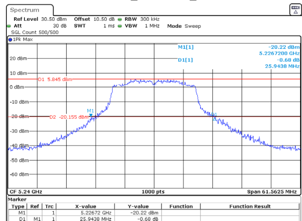
802.11ac20_5240MHz_Chain 1
