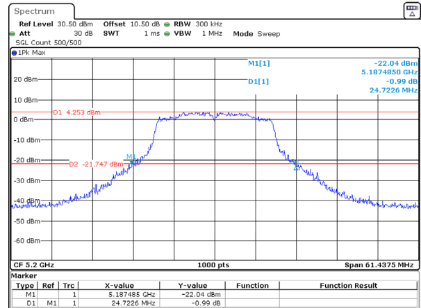
802.11ac20_5200MHz_Chain 0
