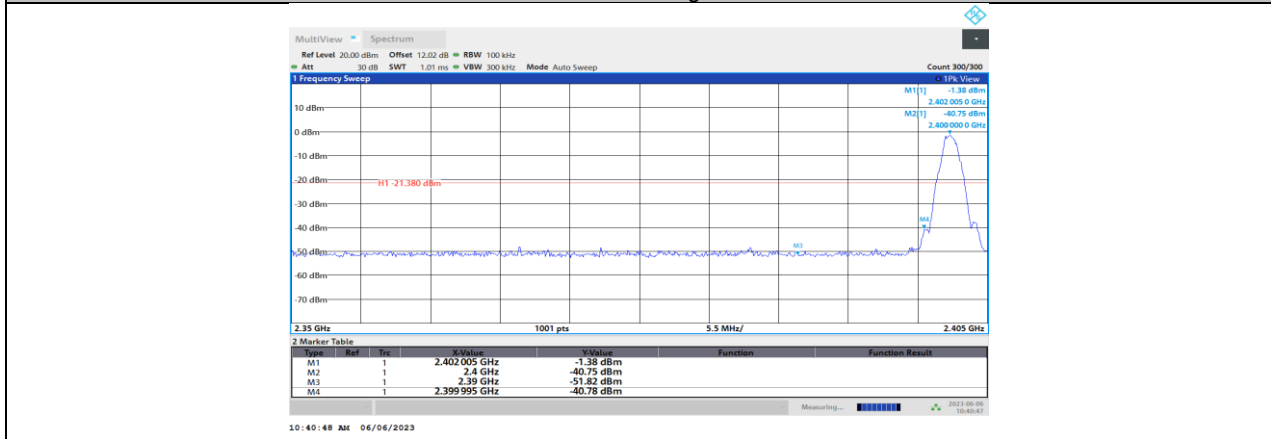
BLE_2M_Ant1_Low_2402
