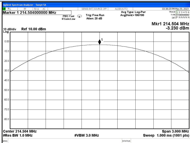
Channel 2 / 214.5MHz
