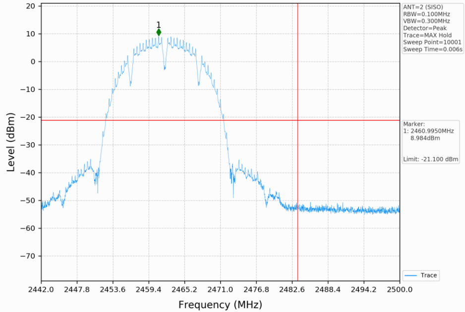
802.11b_2462MHz_SISO_ANT2
