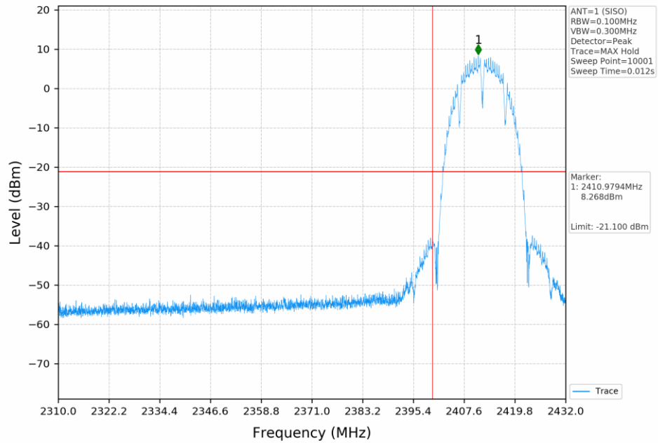
802.11b_2412MHz_SISO_ANT1
