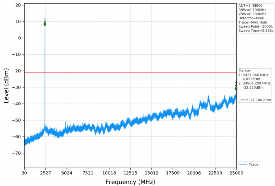
802.11b_2437MHz_SISO_ANT1
