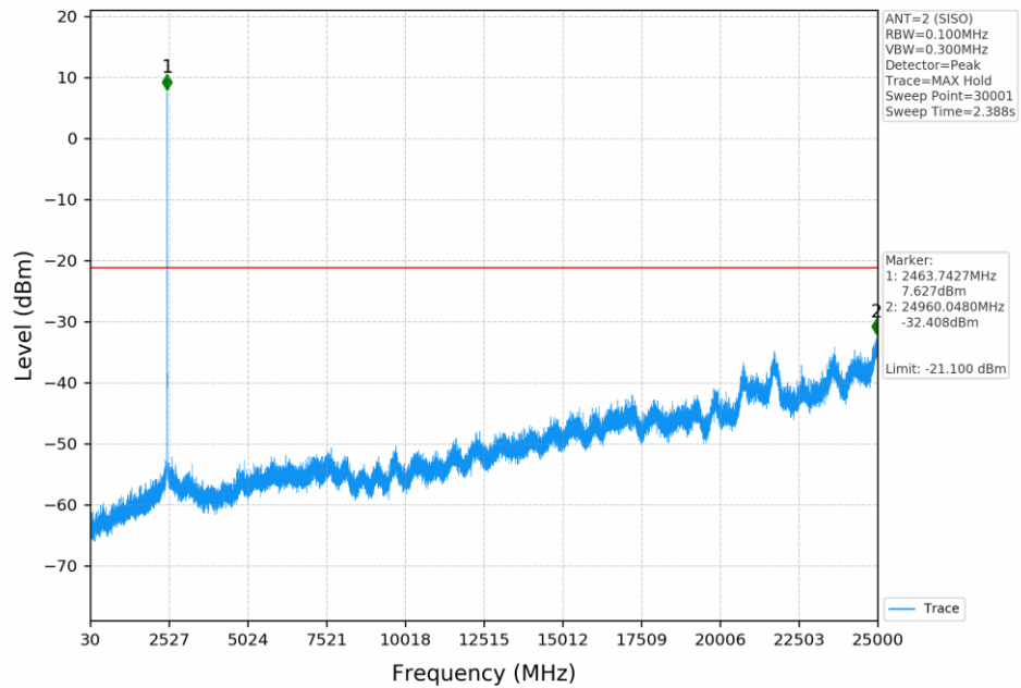
802.11g_SISO_ANT2_REF
