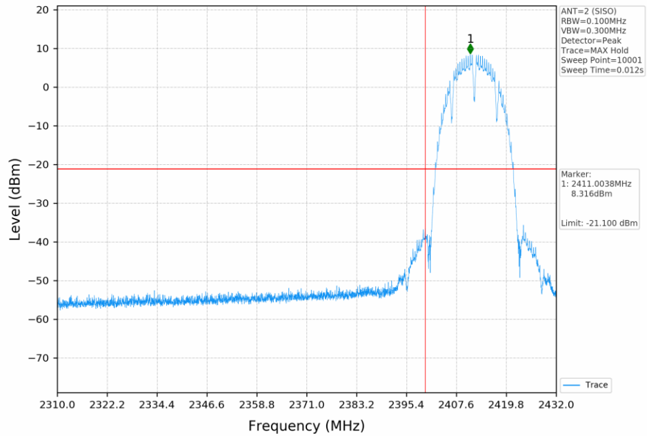
802.11b_2412MHz_SISO_ANT2
