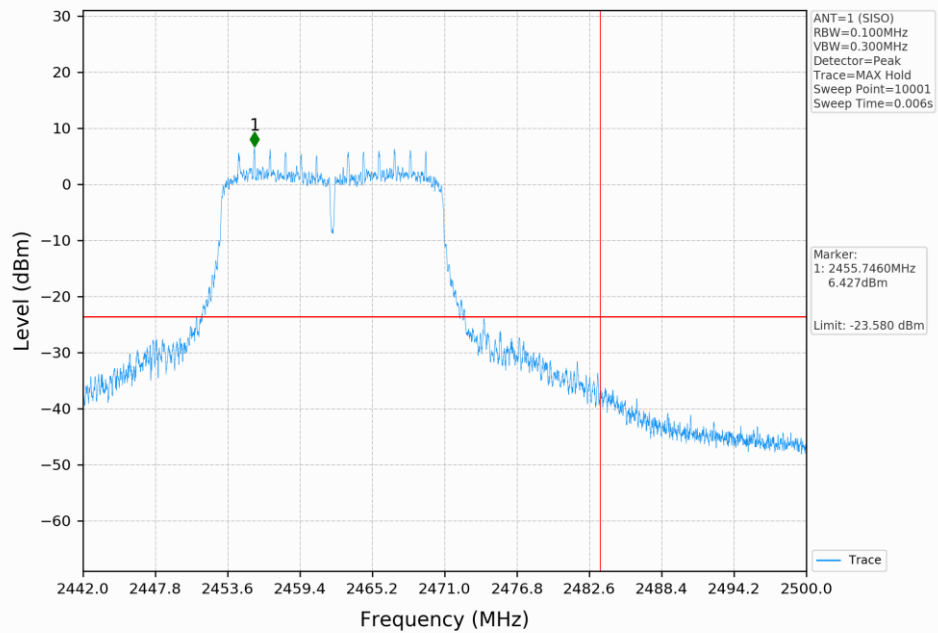
802.11n(HT20)_2462MHz_SISO_ANT1
