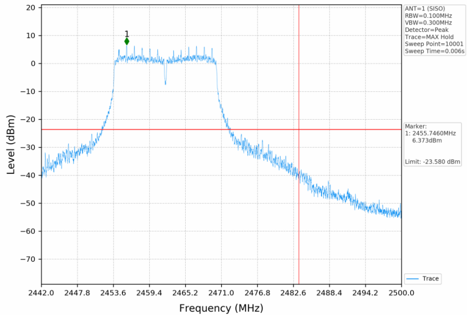
802.11g_2462MHz_SISO_ANT1
