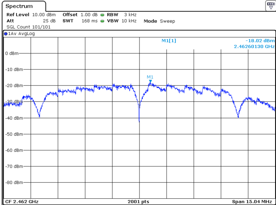
802.11b_2462MHz_SISO_ANT2
