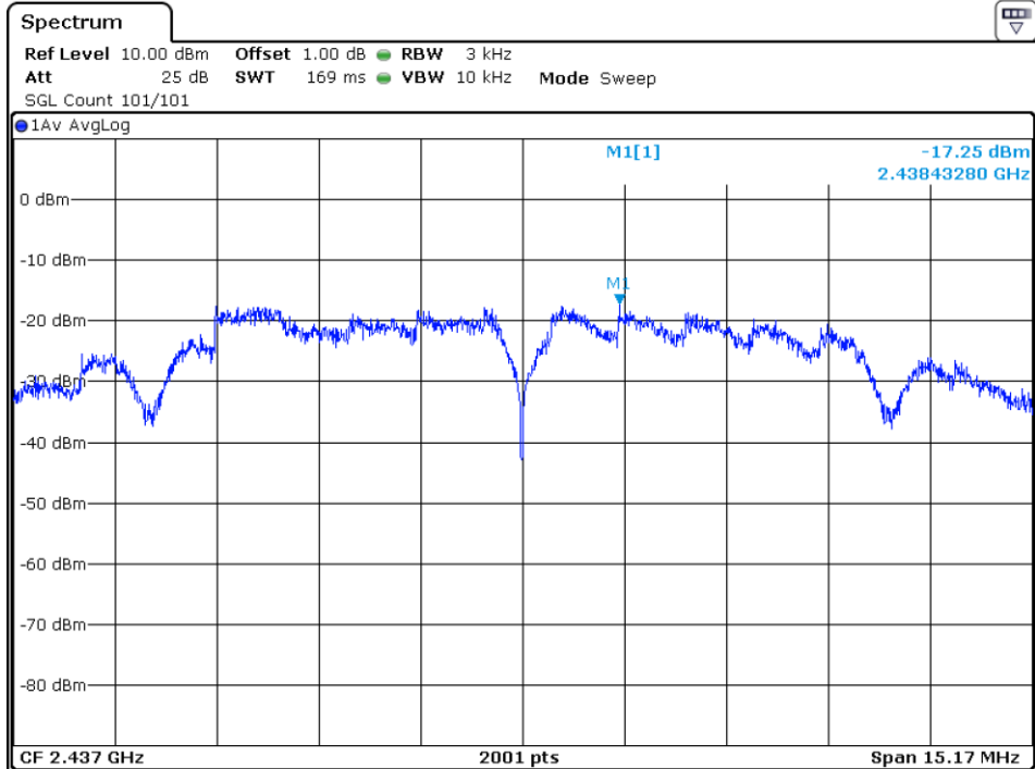
802.11b_2437MHz_SISO_ANT2
