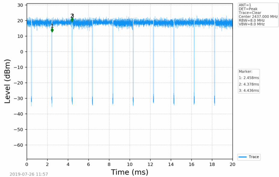
802.11n(HT20)_2437MHz_MIMO_ANT1
