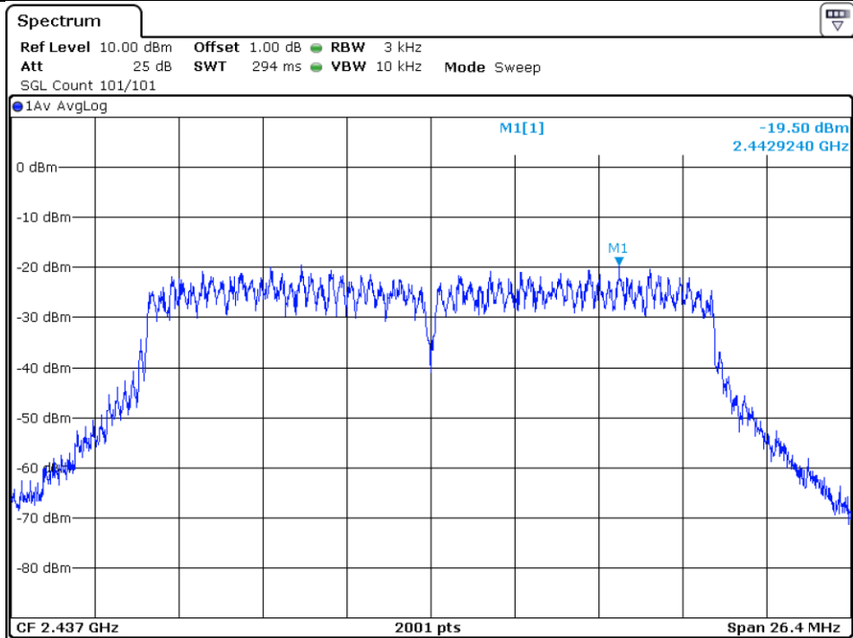
802.11n(HT20)_2437MHz_MIMO_ANT2
