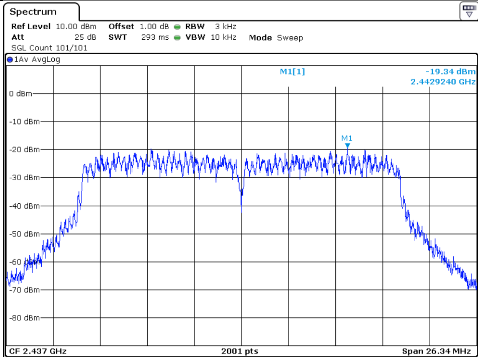
802.11n(HT20)_2437MHz_MIMO_ANT1
