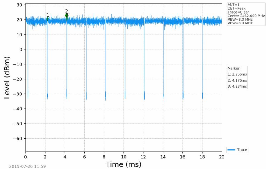
802.11n(HT20)_2462MHz_MIMO_ANT1
