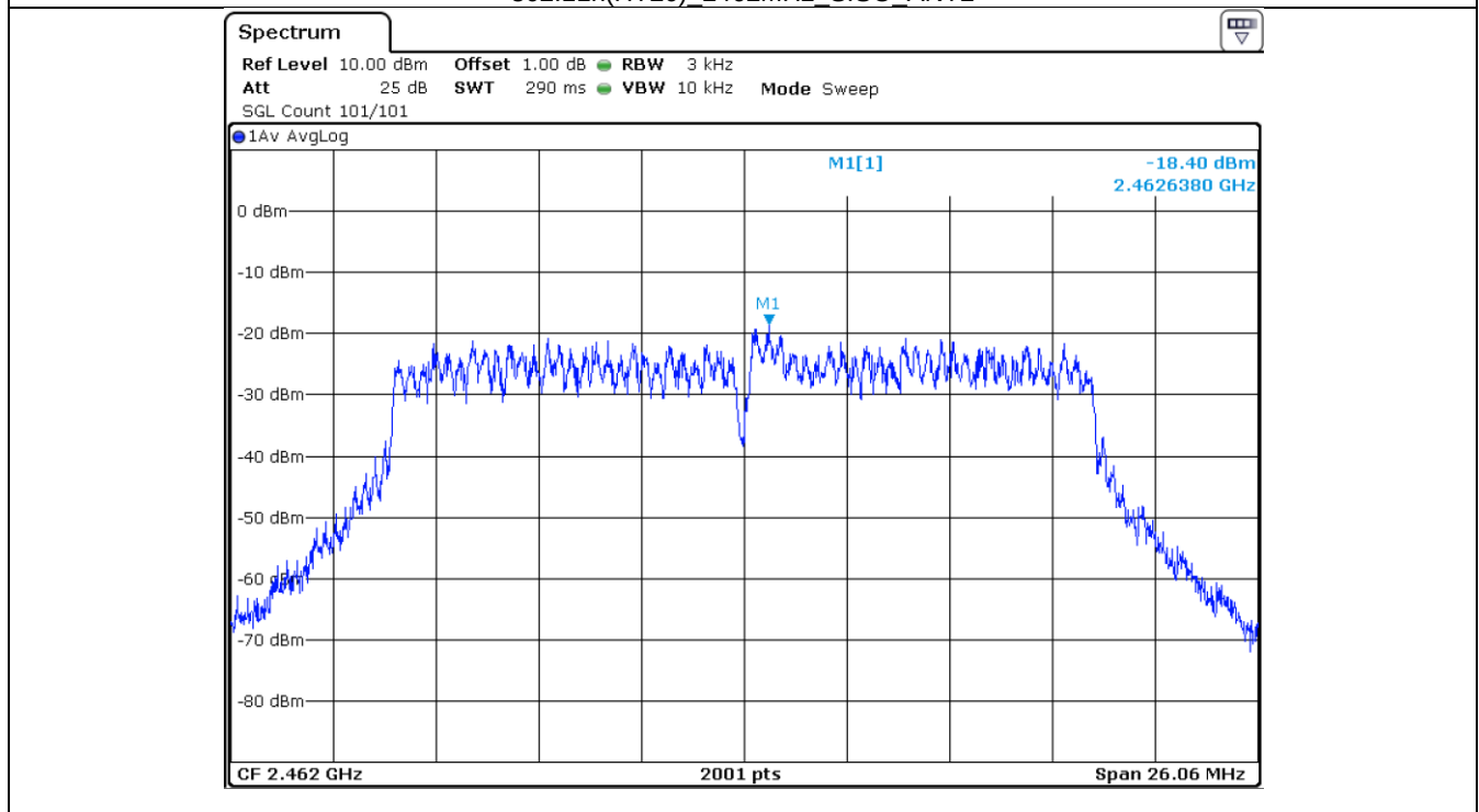
802.11n(HT20)_2462MHz_MIMO_ANT1
