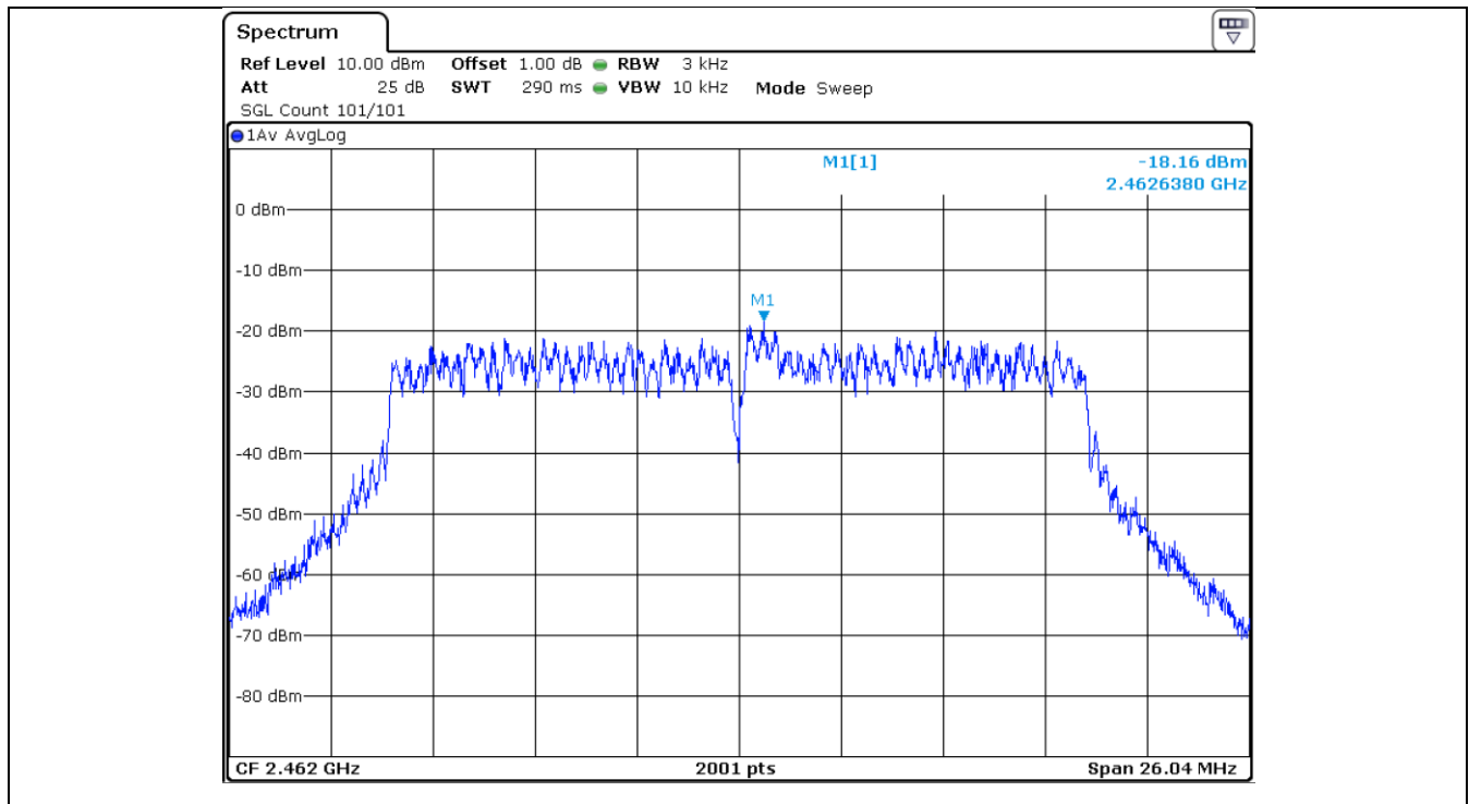
802.11n(HT20)_2462MHz_SISO_ANT2
