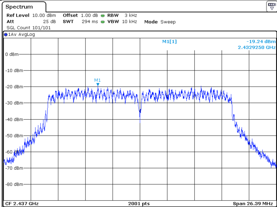
802.11n(HT20)_2437MHz_SISO_ANT2
