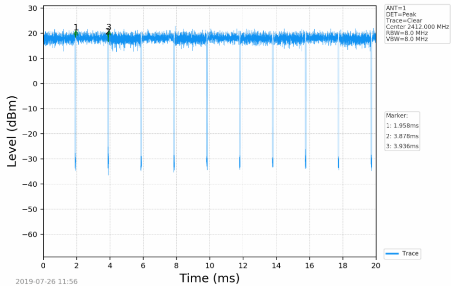
802.11n(HT20)_2412MHz_MIMO_ANT1
