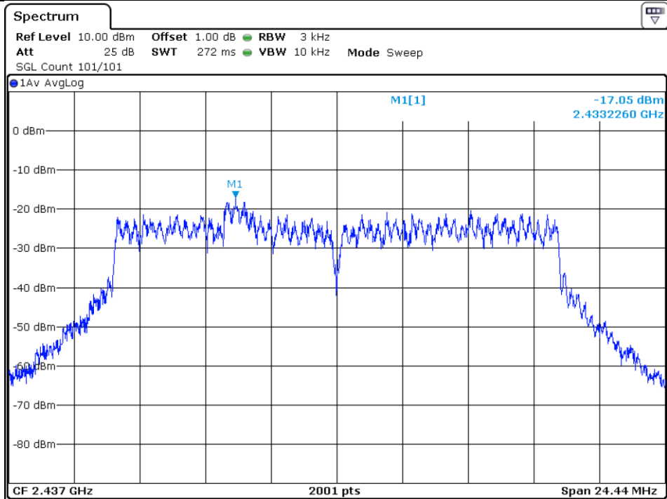
802.11g_2437MHz_SISO_ANT2
