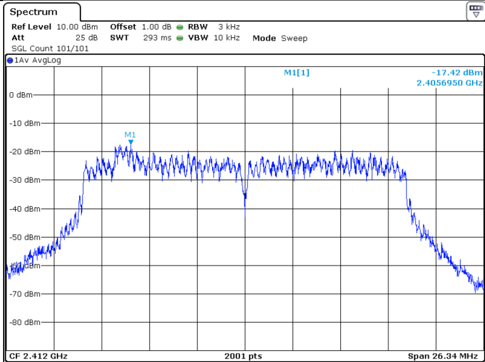
802.11n(HT20)_2412MHz_MIMO_ANT2
