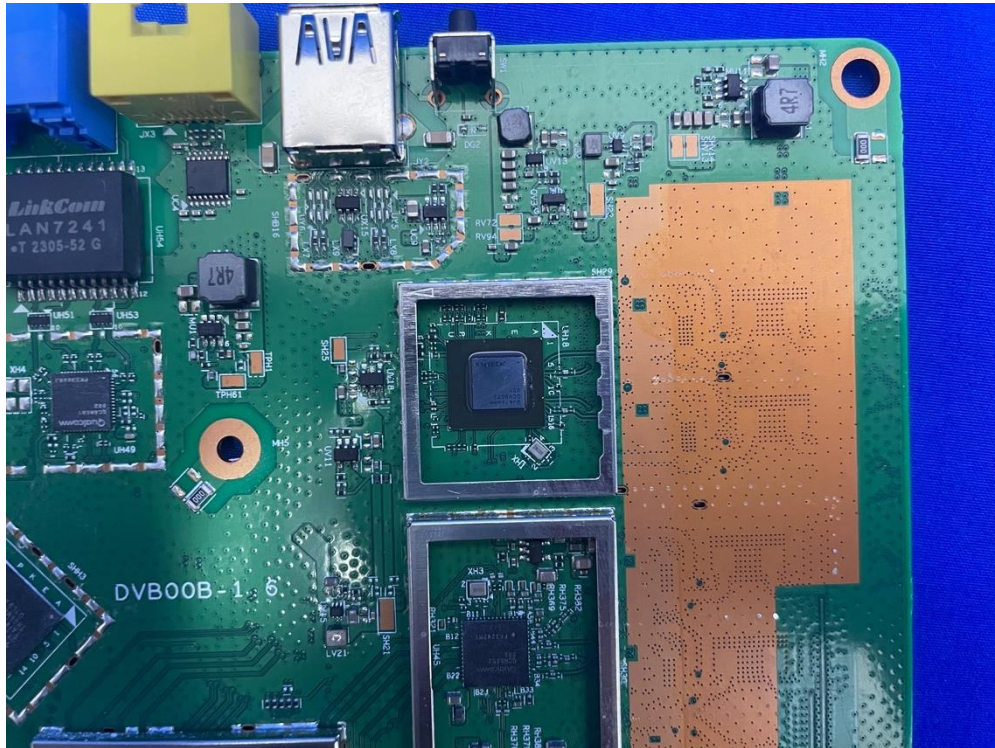
(9) EUT Photo (OAW-AP1431)
