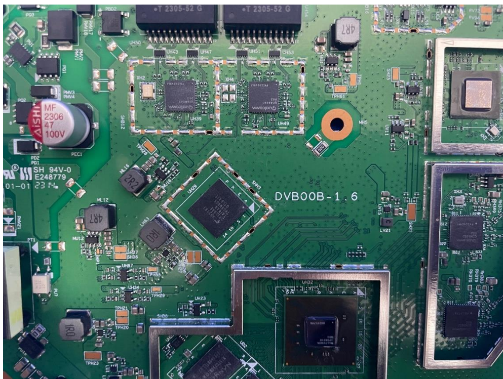
(8) EUT Photo (OAW-AP1431)
