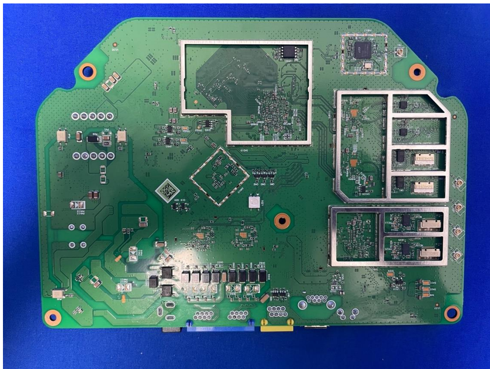
(10) EUT Photo (OAW-AP1431)
