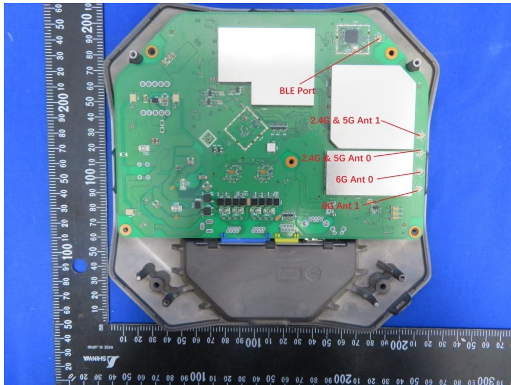
(3) EUT Photo (OAW-AP1431)
