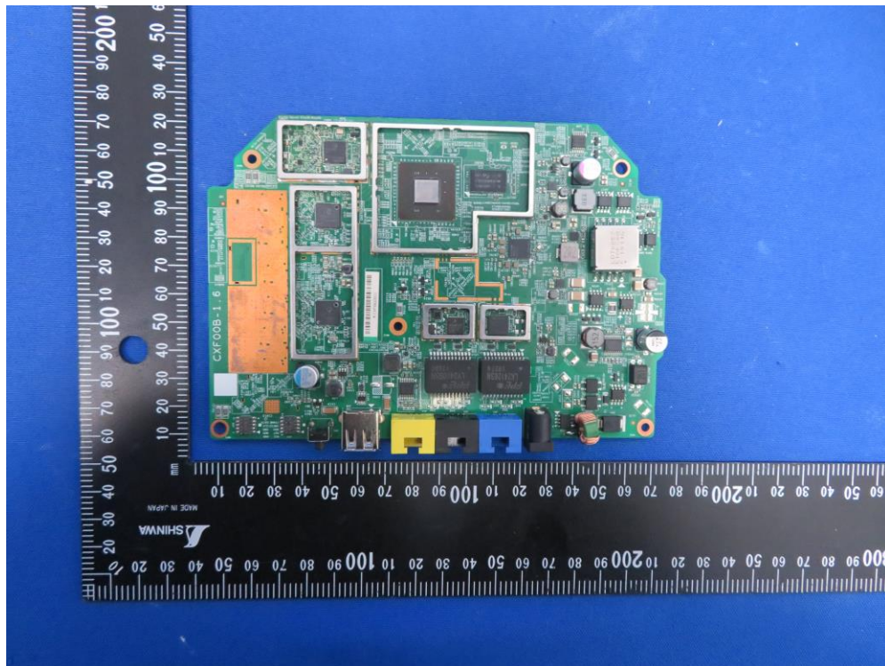
(4) EUT Photo_OAW-AP1321
