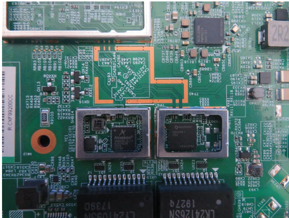
(7) EUT Photo_OAW-AP1321
