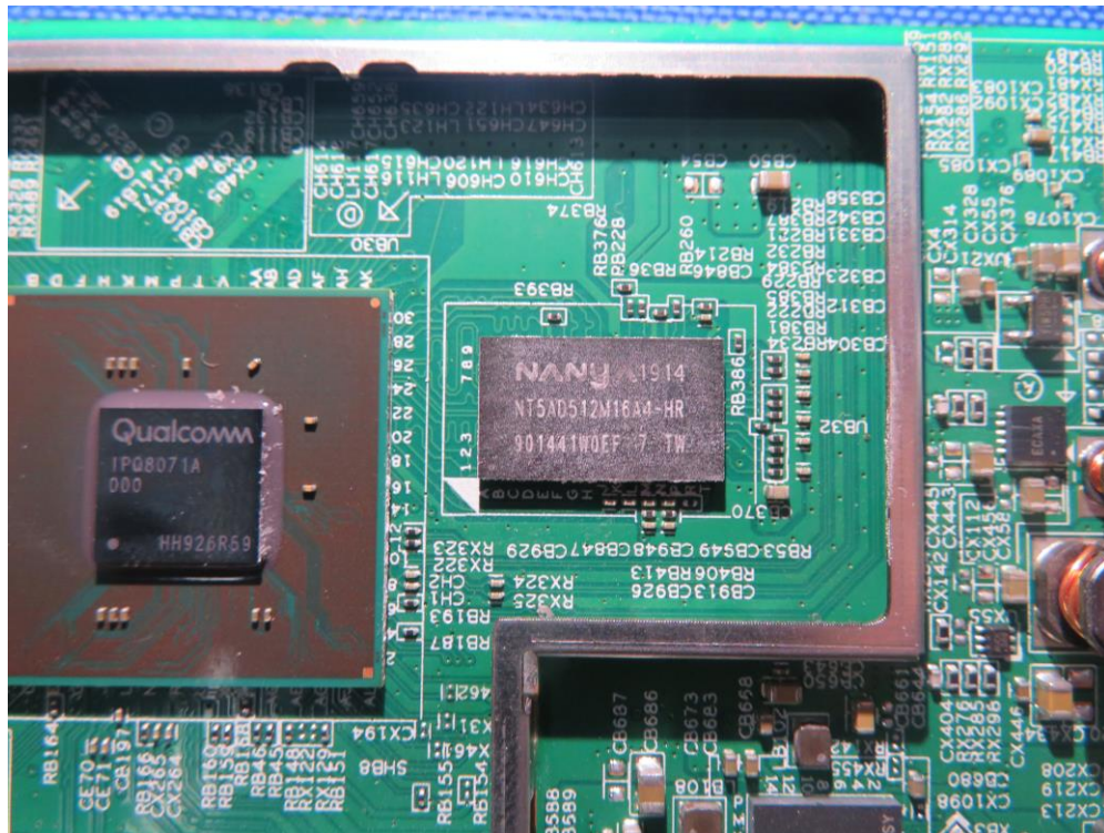
(5) EUT Photo_OAW-AP1321
