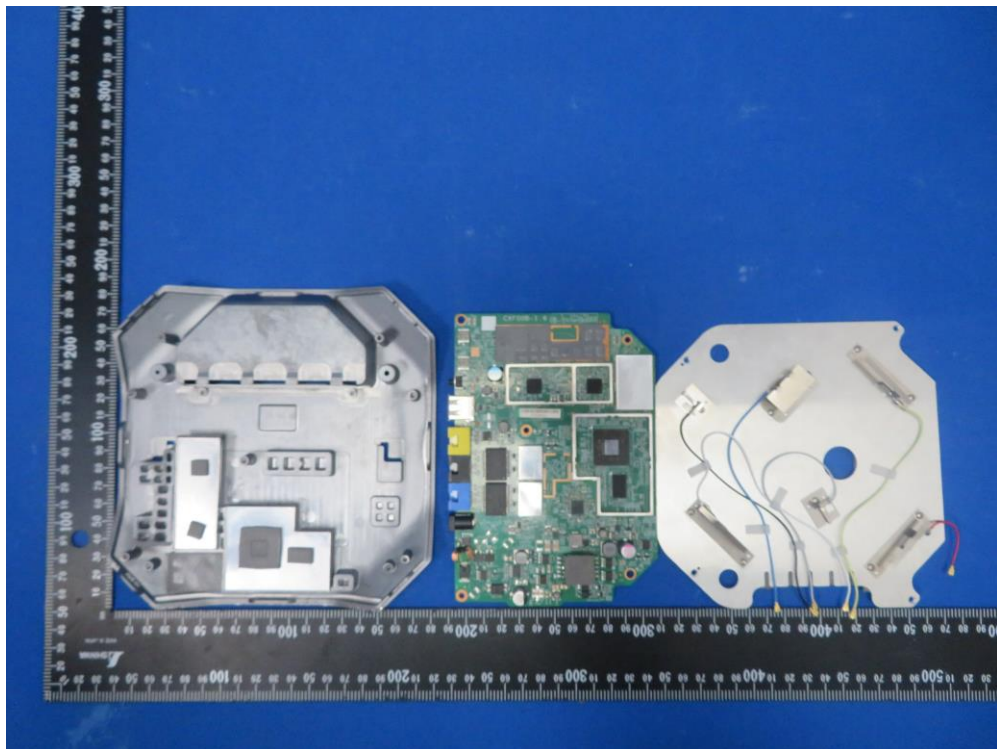
(2) EUT Photo_OAW-AP1321
