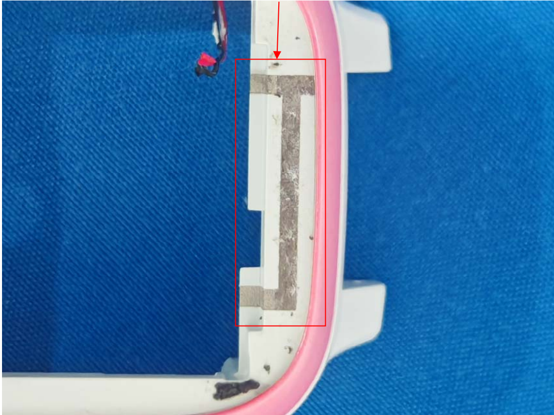
WWAN Antenna
