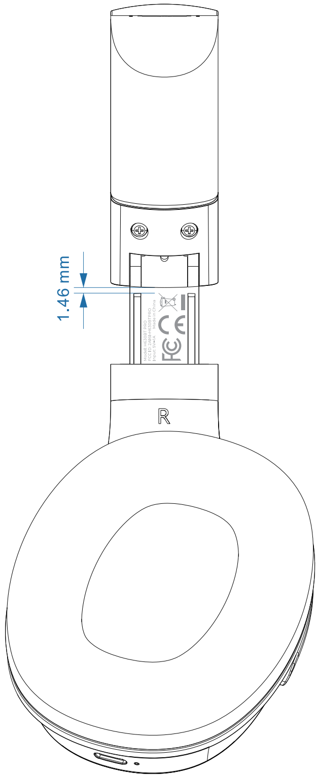
右支臂内侧
