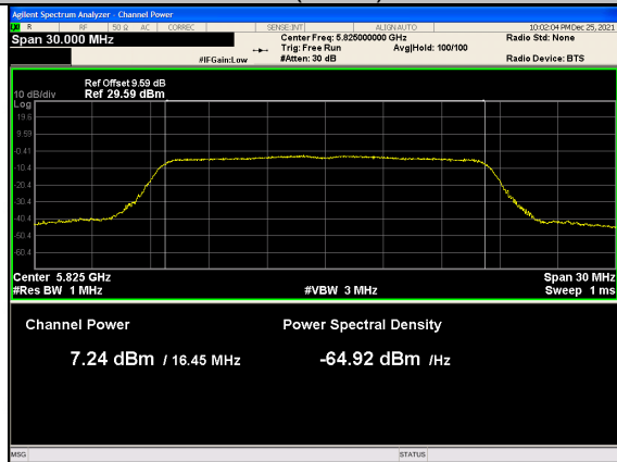
802.11ac(VH20)-5825
