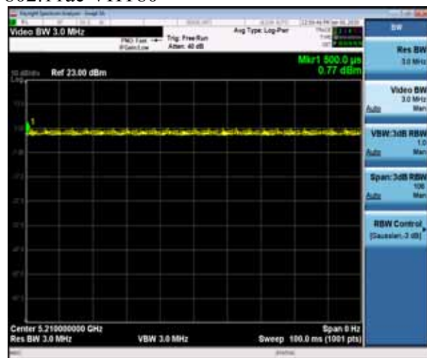
802.11ac VHT80
