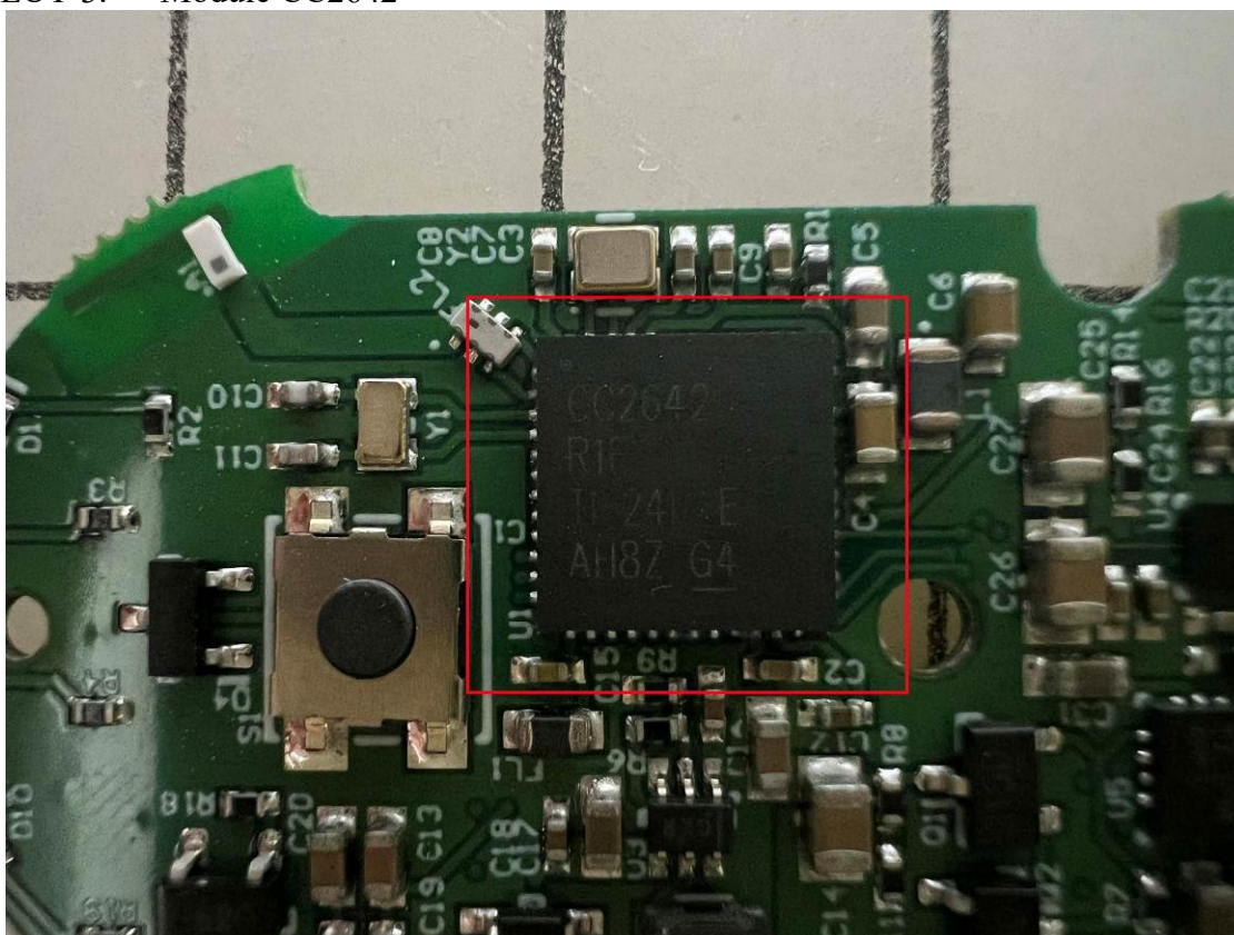
EUT-3. Module CC2642
