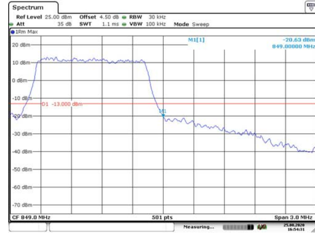
1.4M, 16QAM, Right Band Edge
