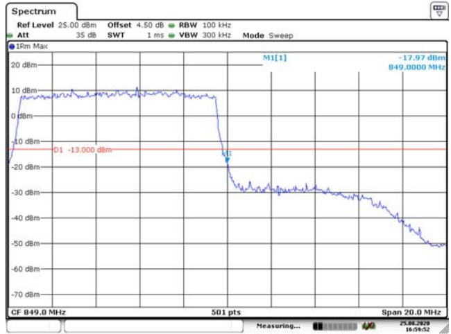
10M, QPSK, Right Band Edge
